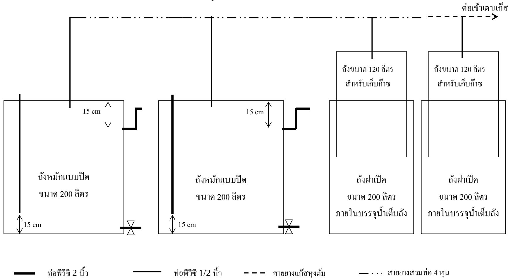
ภาพที่ 9 รูปแบบการก่อสร้างระบบการบำบัดน้ำเสียจากการผลิตปลาตู้ร่ำ ด้วยการหมักแบบไร้อากาศ ณ ครัวเรือนนาร่อง
