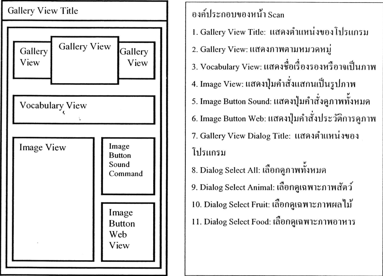
รูปที่ ก.37 User Interface : Gallery System Design
