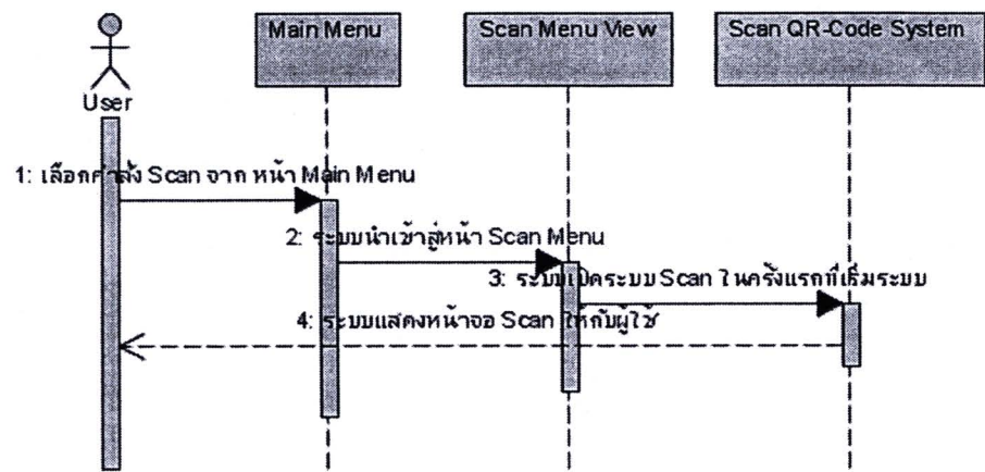
รูปที่ ก.17 UML Sequence Diagram : Scan Menu System
