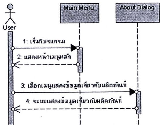
รูปที่ ๓.31 UML Sequence Diagram : About System
