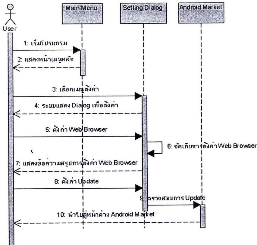
รูปที่ ๓.30 UML Sequence Diagram : Setting System
