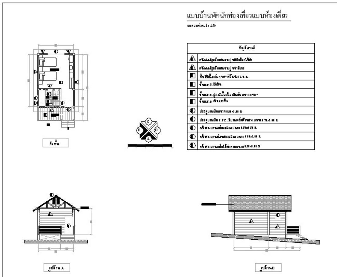
ภาพผนวกที่ 1 แบบบ้านพักนักท่องเที่ยวแบบห้องเดี่ยว
