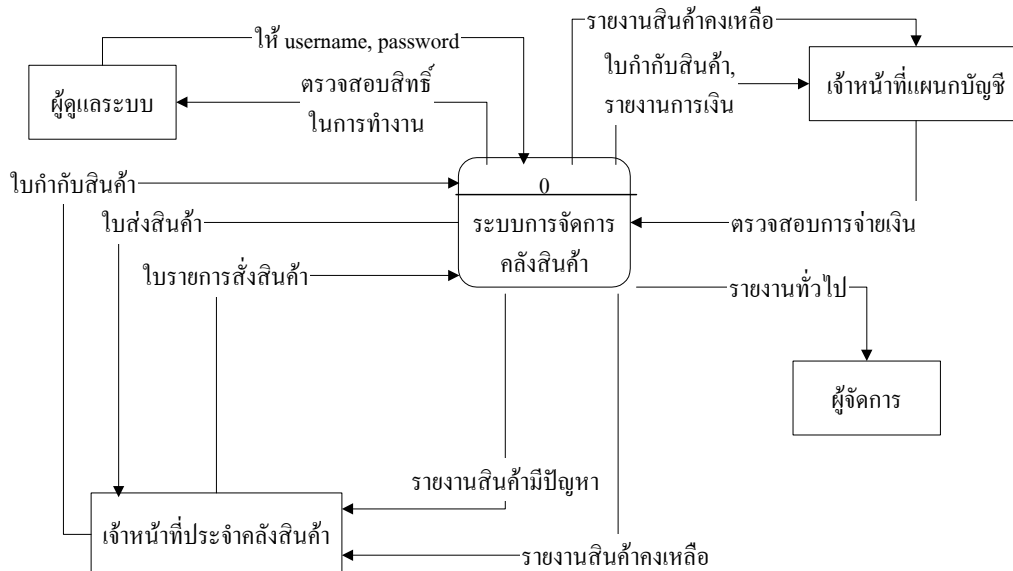
รูป 4.1 แผนภาพบริบทของระบบ
