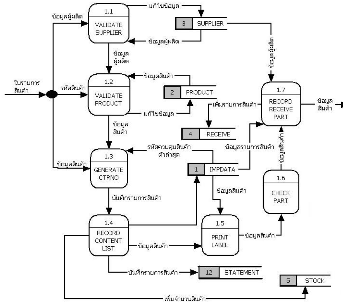
รูป 4.3 แผนภาพกระแสการไหลของข้อมูล ระดับที่ 1 ของกระบวนการที่ 1
