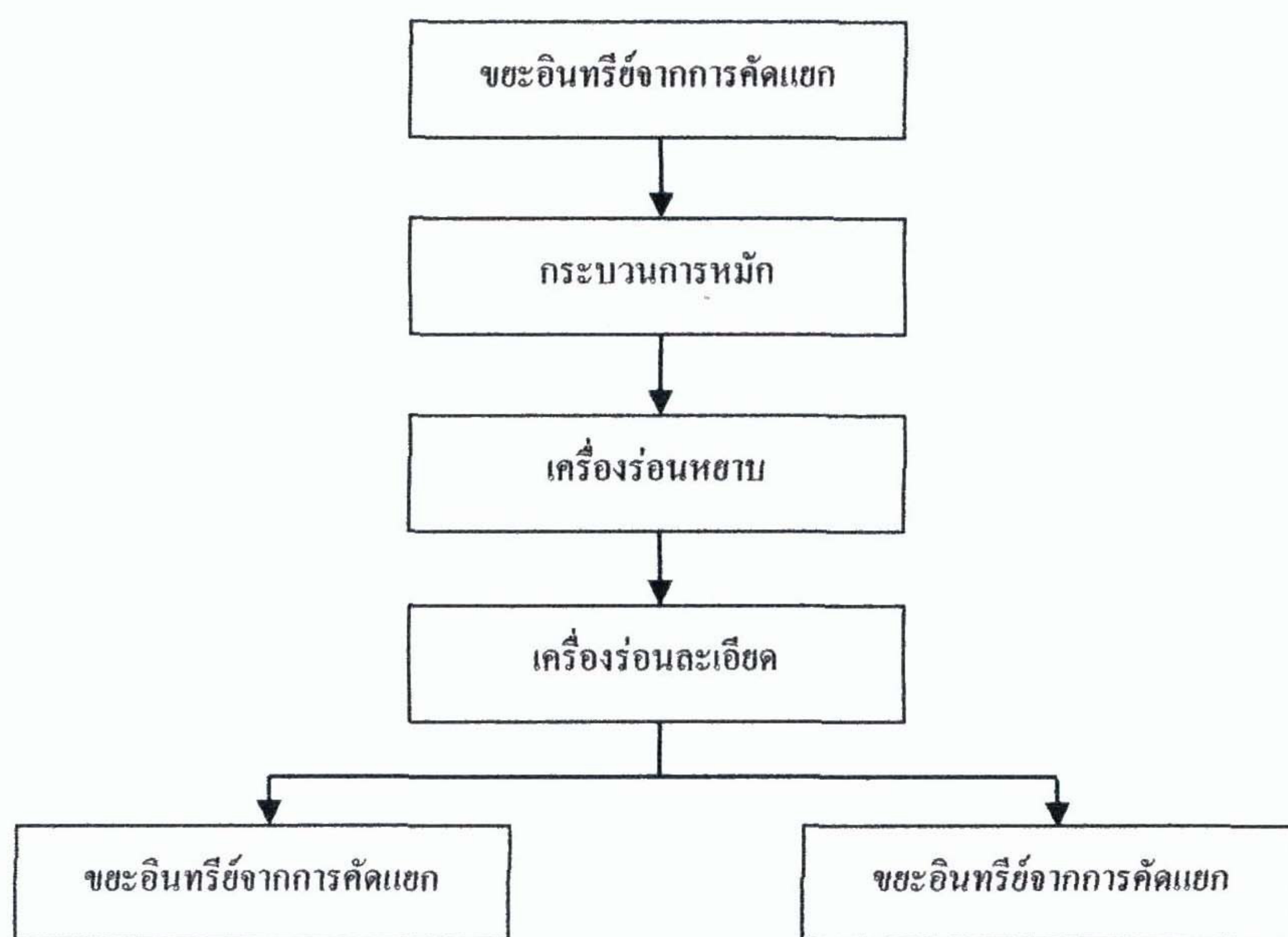
รูปที่ 2.1-11 ระบบหมักปุ๋ยของเทศบาลตำบลเวียงฝาง
