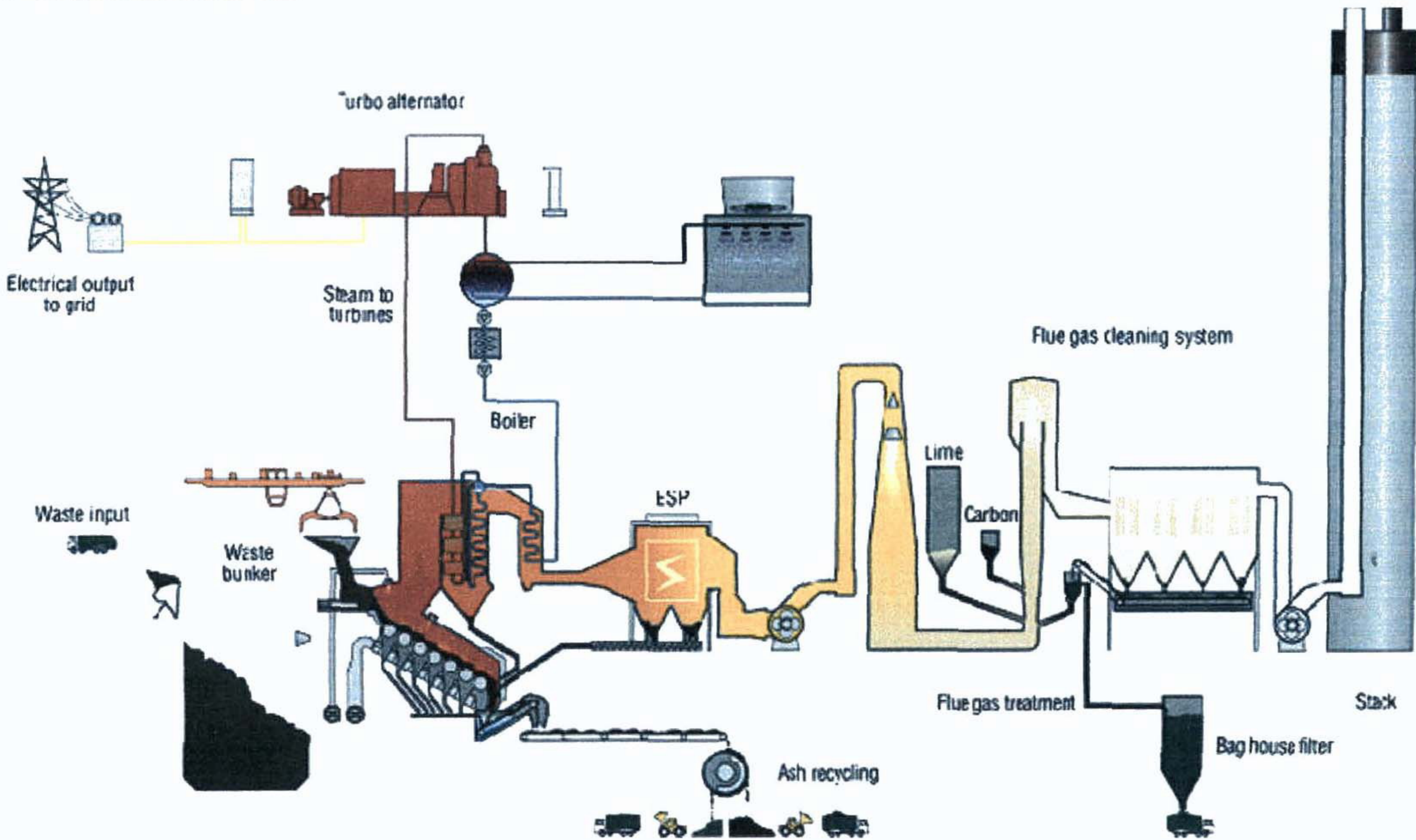
รูปที่ 2.2-2 ระบบผลิตพลังงานจากขยะมูลฝอยด้วยเทคโนโลยีเตาเผามูลฝอย
