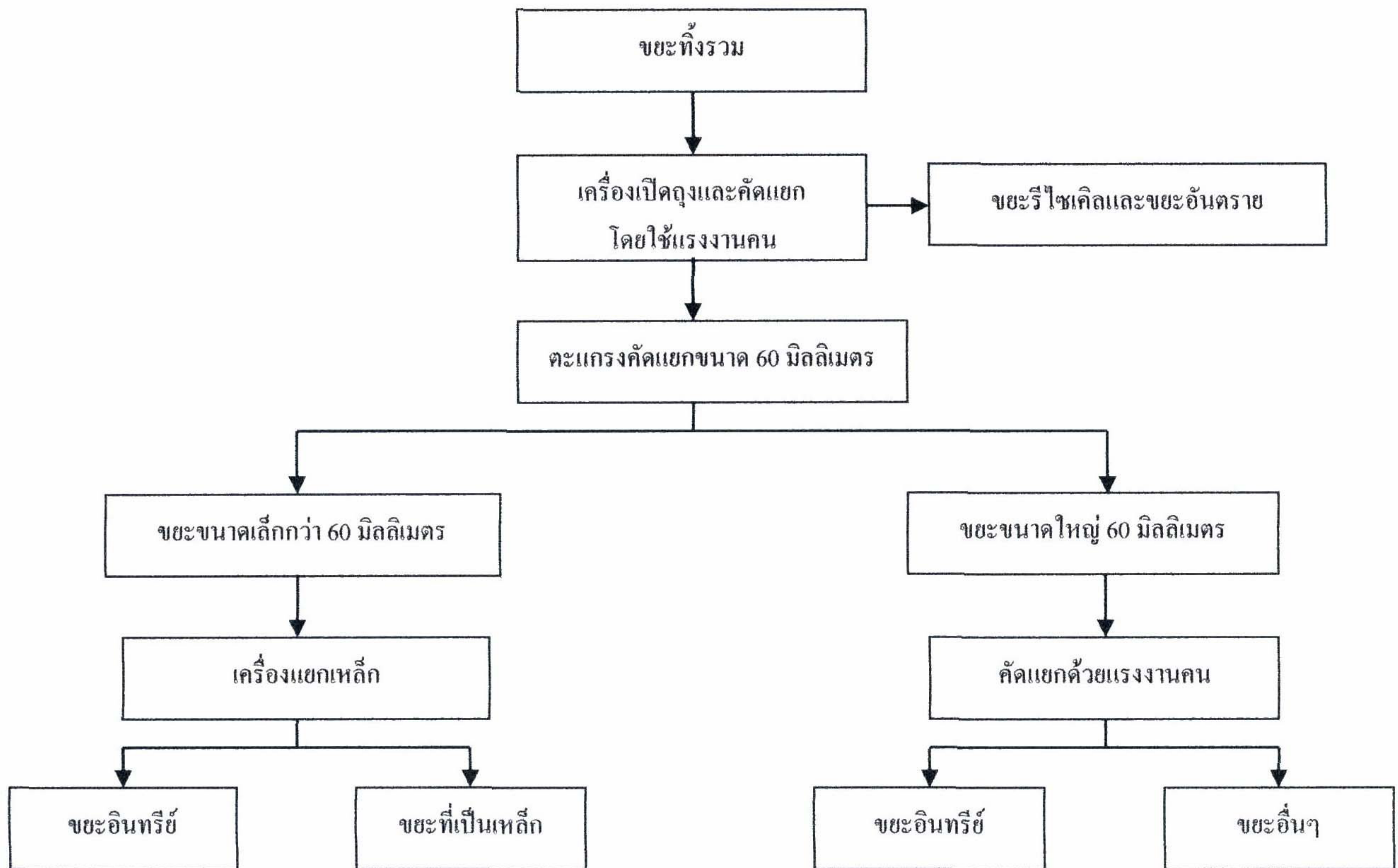
รูปที่ 2.1-5 กระบวนการคัดแยกขยะทิ้งรวมของเทศบาลนครระยอง
