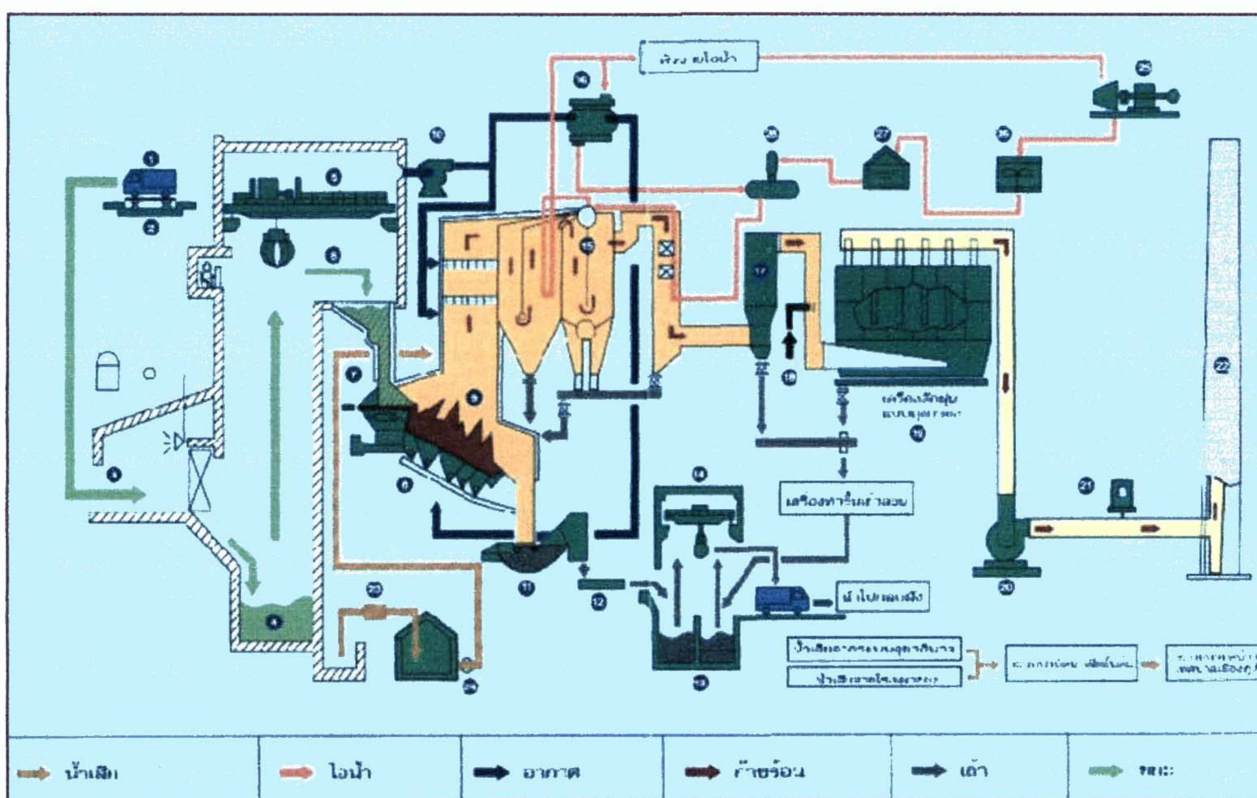
รูปที่ 2.1-2 แผนผังพื้นที่และการทำงานของเตาเผาขยะมูลฝอยของจังหวัดภูเก็ต (ศูนย์วิจัยการเผากากของเสีย, 2551)
