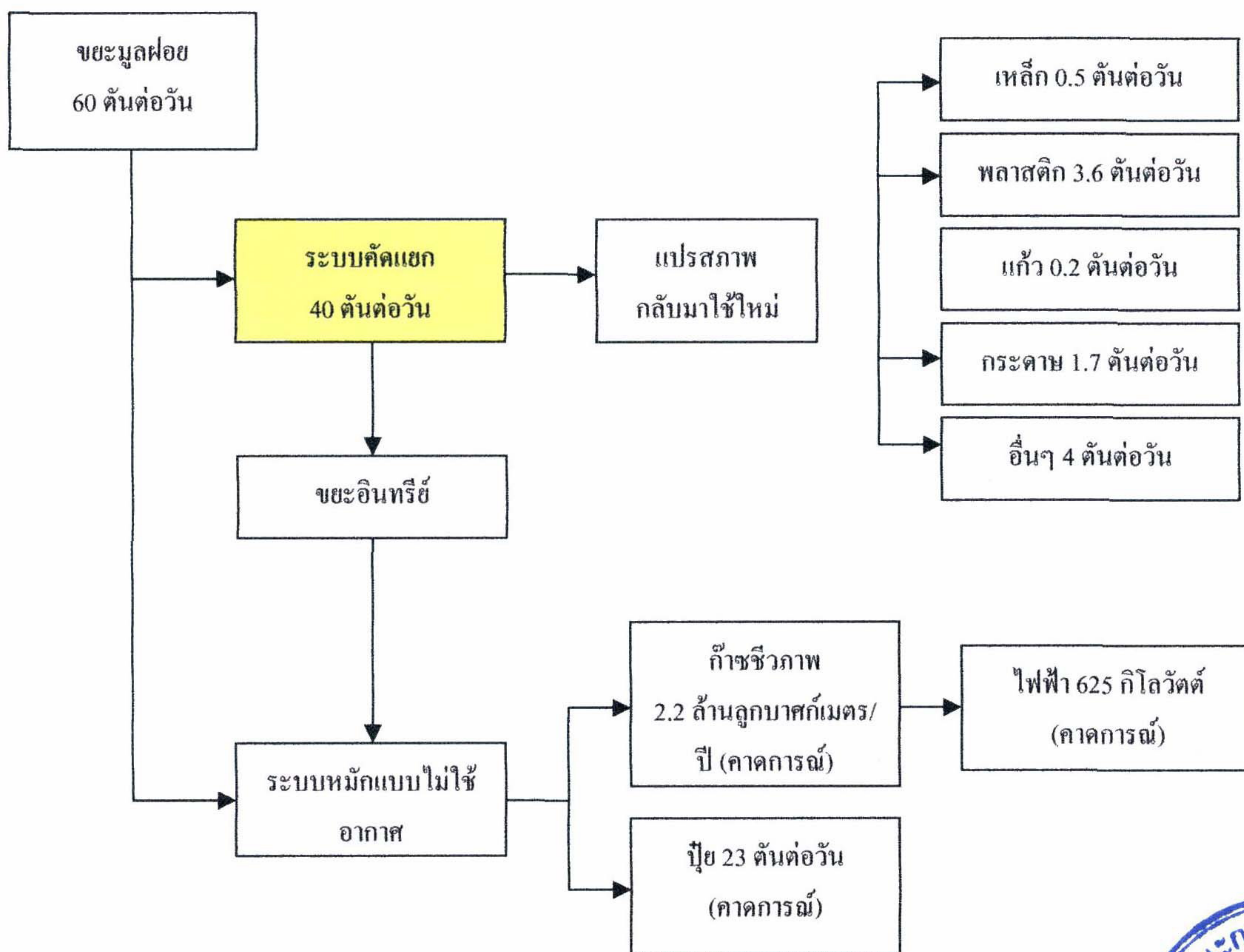
รูปที่ 2.1-3 ภาพรวมการจัดการขยะมูลฝอยของเทศบาลนครระยอง
