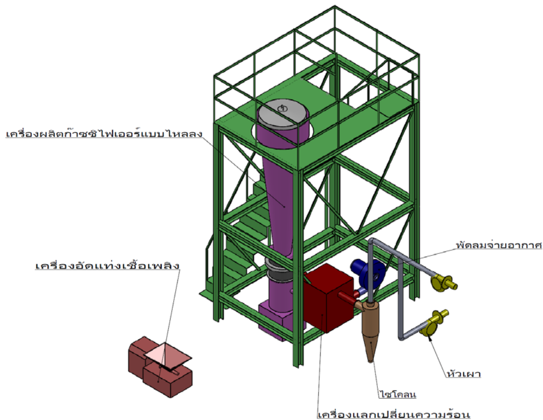
รูปที่ 4.4-12 องค์ประกอบของระบบก๊าซซิฟเออร์แบบไหลลง
