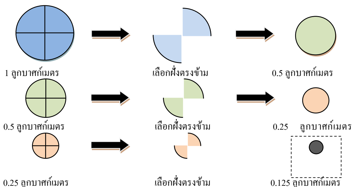
รูปที่ 3.1-7 ลำดับขั้นตอนการ Quartering (ธีเรศ, 2553)
