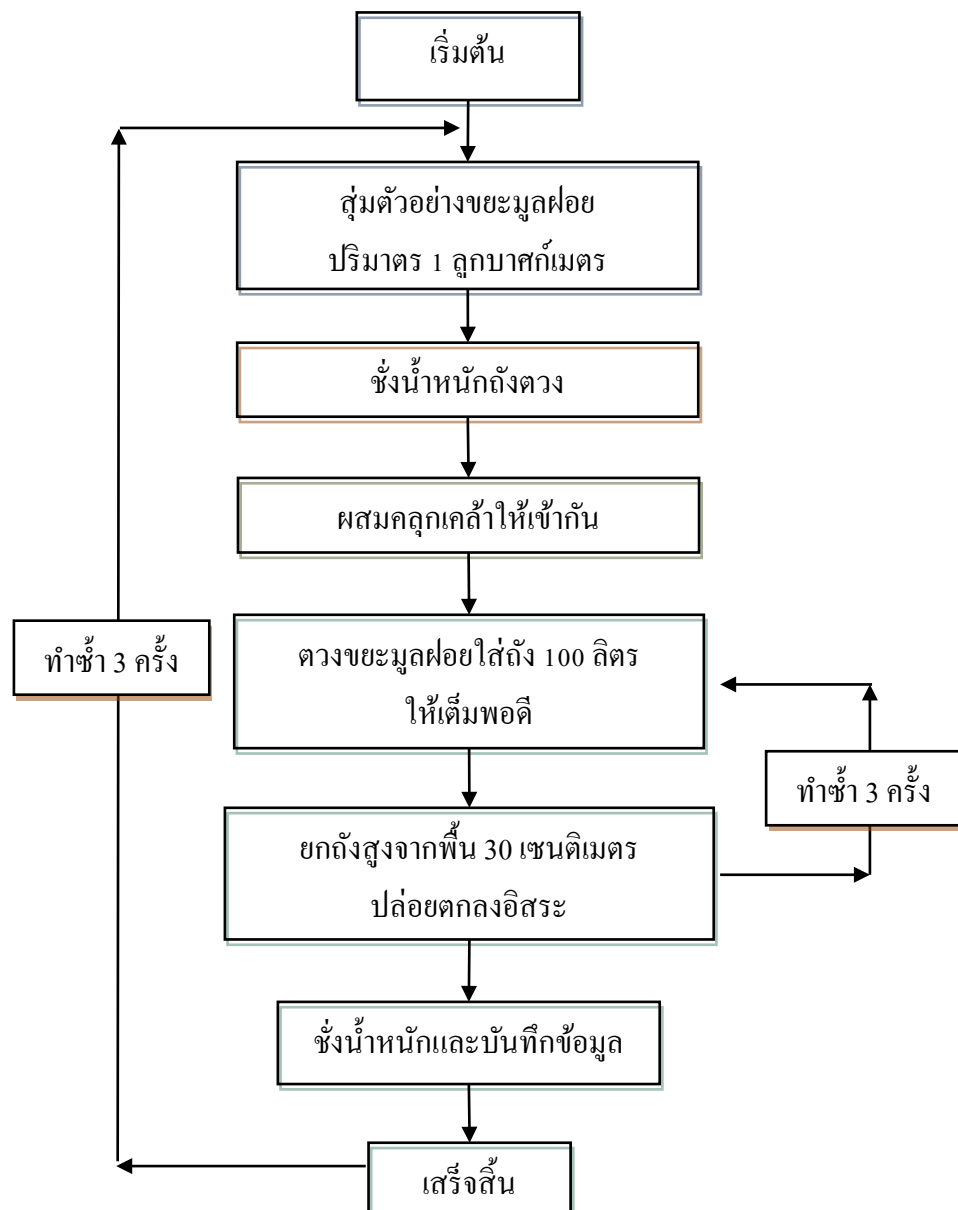
รูปที่ 3.1-6 ขั้นตอนการวัดค่าความหนาแน่นขยะมูลฝอย (ชเรศ, 2553)
