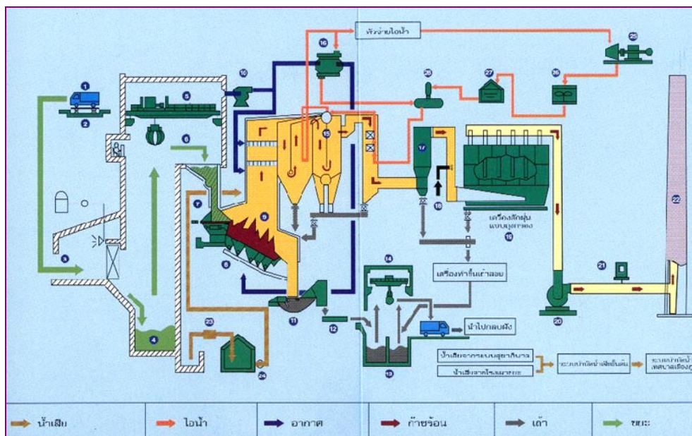
รูปที่ 2.1-2 แผนผังพื้นที่และการทำงานของเตาเผาขยะมูลฝอยของจังหวัดภูเก็ต
