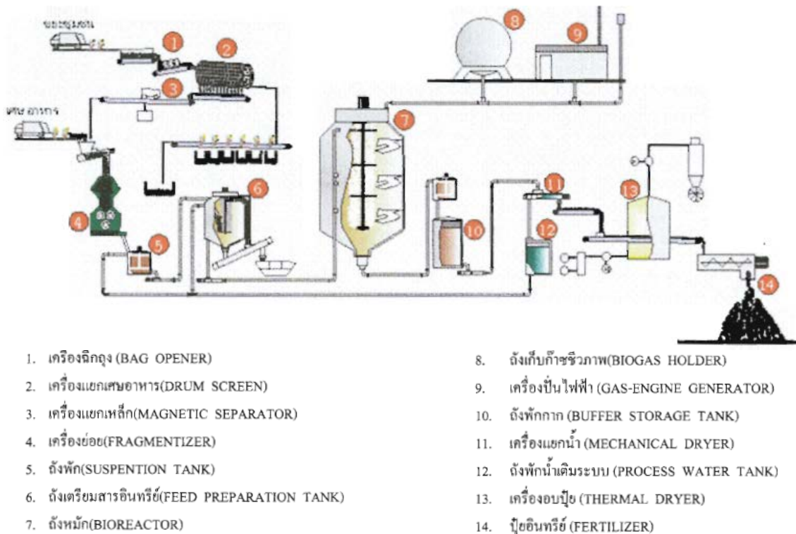
รูปที่ 2.1-4 เครื่องจักรและอุปกรณ์หลักของระบบกำจัดขยะมูลฝอยเทศบาลนครระยอง (เสรีย์, 2548)
