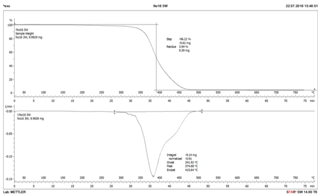
ภาพที่ 39 โคโรมาโตรแกรม TGA ของชิ้นงานตัวอย่างยาง WEEK 3
