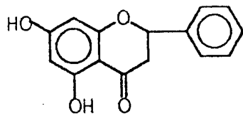
pinocembrin (1)
