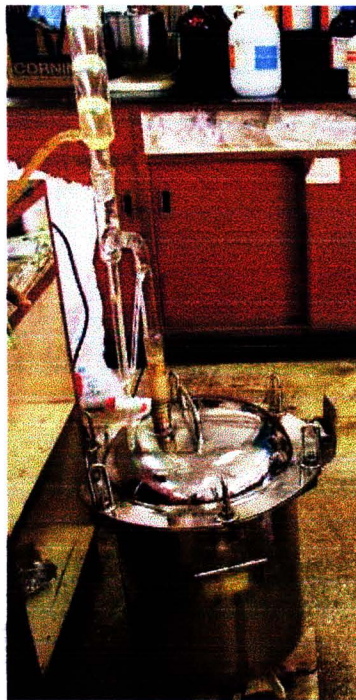
รูปที่ 2-2 แสดงการกลั่นน้ำมันหอมระเหยในภาชนะกลั่นแบบ 10 ลิตร
