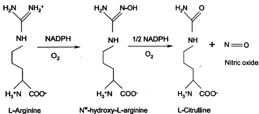
รูปที่ 2-2 ปฏิกิริยาการสังเคราะห์ไนตริกออกไซด์โดยเอนไซม์ NOS
