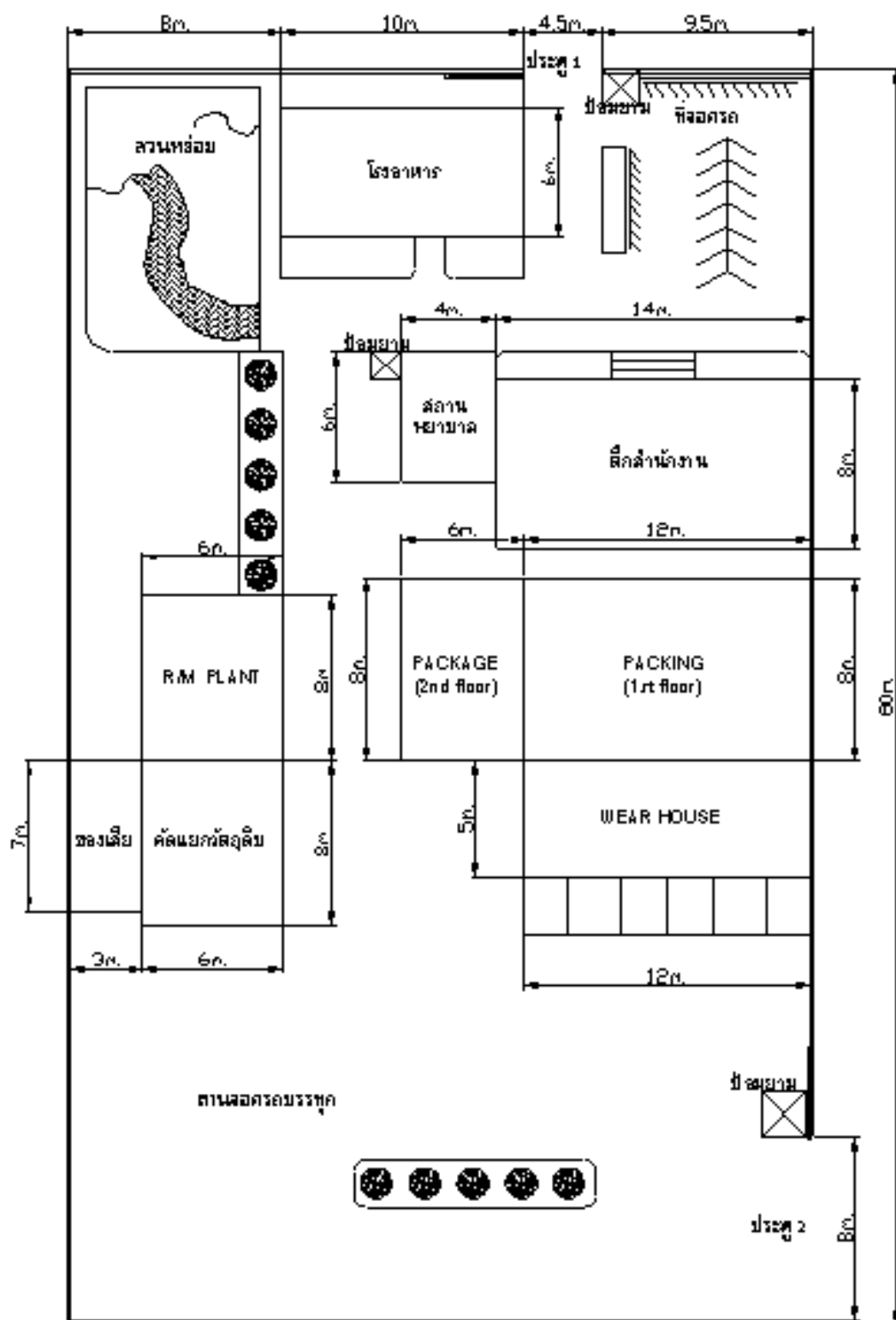
ภาพผนวกที่ 1 แบบผังโรงงานผลิตเม็ดพลาสติกจากขยะพลาสติกเชิงซ้อน
