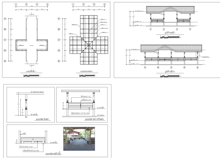
ภาพที่ 3.3-1 การรังวัดศาลาทำน้ำ
