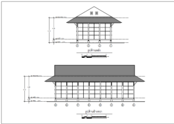
ภาพที่ 3.5-1 การรังวัดยั้งช้า
