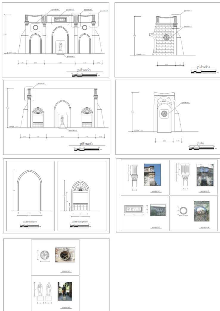
ภาพที่ 3.6-2 การรังวัดโบสถ์เก่า
