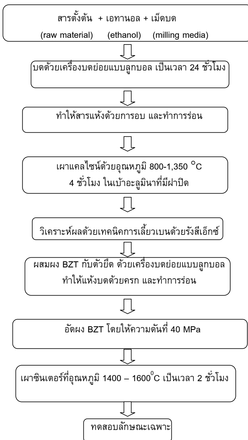
ภาพ 23 ขั้นตอนการเตรียมเซรามิกแบเรียมเซอร์โคเนตไททาเนต โดยวิธีการปฏิกิริยาสถานะของแข็ง
