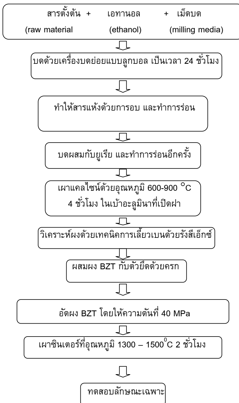
ภาพ 24 ขั้นตอนการเตรียมเซรามิกแบเรียมเซอร์โคเนตไททาเนตโดยวิธีการเผาใหม่
