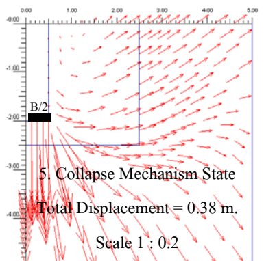
ภาพผนวกที่ ข4 เวกเตอร์การเคลื่อนตัวของดินทราย กรณีที่ D/B = 2
