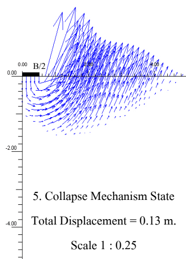
ภาพผนวกที่ ข5 Total Incremental Displacement ของ Medium Sand กรณีที่ D/B = 0
