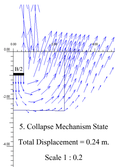
ภาพผนวกที่ ข7 Total Incremental Displacement ของ Medium Sand กรณีที่ D/B = 1
