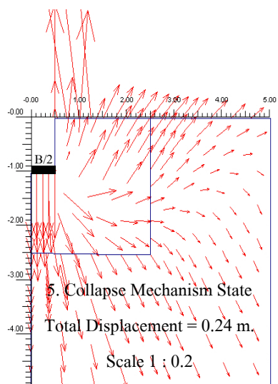
ภาพผนวกที่ ข3 เวกเตอร์การเคลื่อนตัวของดินทราย กรณีที่ D/B = 1
