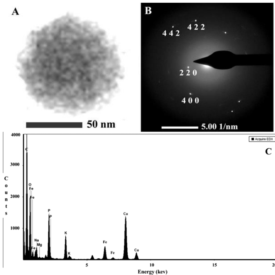
ภาพที่ 4.18 ลักษณะทางกายภาพ องค์ประกอบของแร่ธาตุ และโครงสร้างผลึกออกไซด์ของเหล็กของอนุภาคหลังจากการเผาเซลล์แบคทีเรีย Acinetobacter sp. HER_I ที่อุณหภูมิสูง โดยภาพ A แสดงลักษณะทาง
