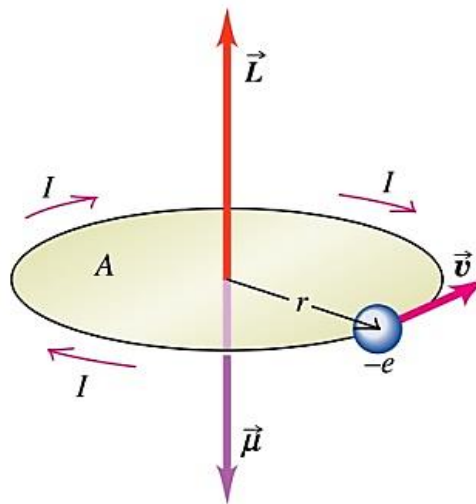
ภาพที่ 2.1 การจำลองแมกนีติกไดโพลโมเมนต์ (Callister and Rethwisch, 2011)
