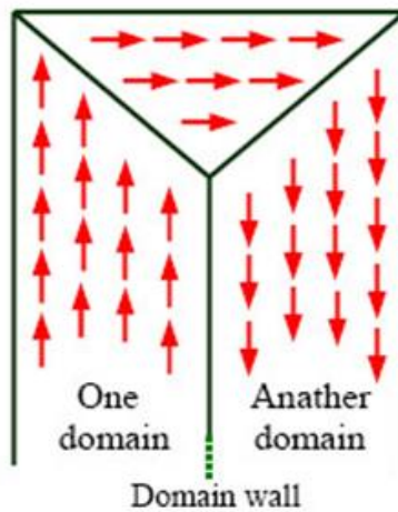
ภาพที่ 2.4 โดเมนแม่เหล็กและทิศทางของไดโพลโมเมนต์แม่เหล็กในแม่เหล็กแบบเฟอร์โรแมกเนติก (Chambers et al., 2006)
