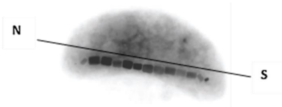
ภาพที่ 2.12 ลักษณะแมกนีโตโซมเรียงต่อเป็นสายตามแนวสนามแม่เหล็ก จากกล้องจุลทรรศน์อิเล็กตรอนแบบส่องผ่าน โดย N = แม่เหล็กขั้วเหนือ S = แม่เหล็กขั้วใต้ (Molcan et al., 2017)
