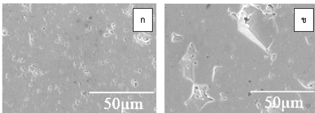
รูปที่ 4.6 โครงสร้างจุลภาคของชิ้นงานอะลูมินาที่ผ่านการเผาที่อุณหภูมิ (ก) 1600 องศาเซลเซียส (ข) 1700 องศาเซลเซียส
