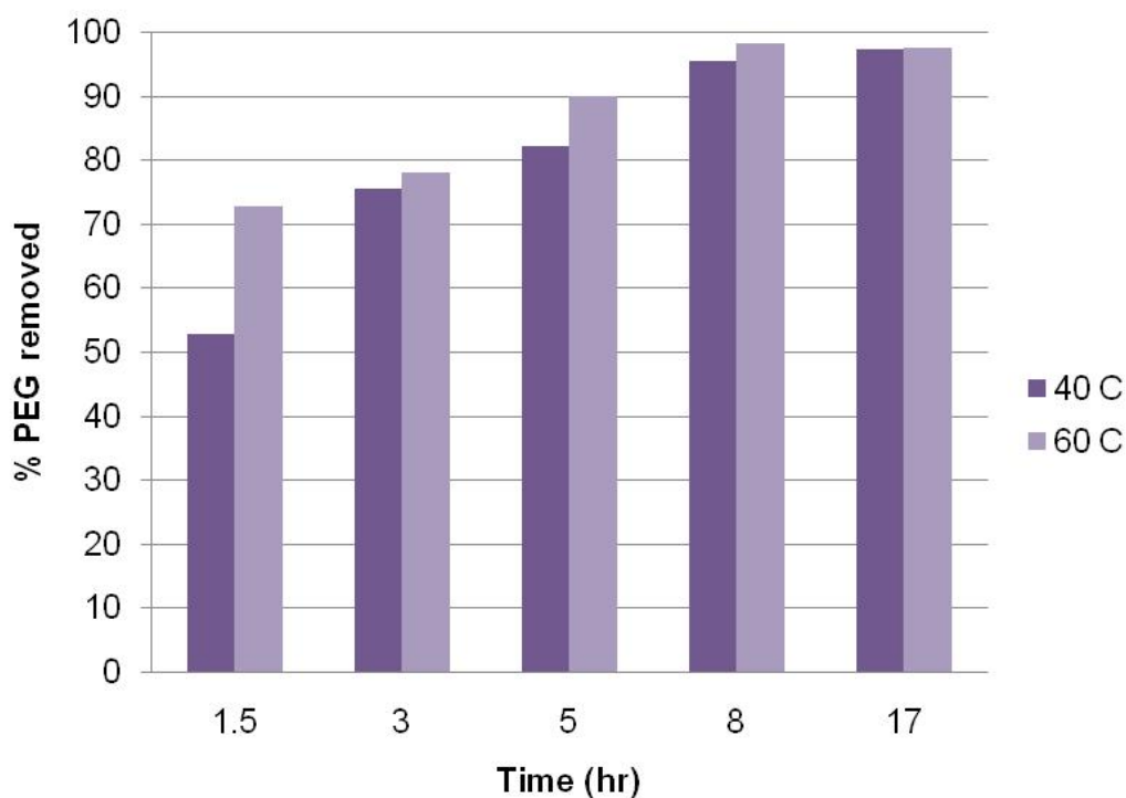
รูปที่ 4.5 กราฟแสดงร้อยละตัวประสานชนิด PEG ที่ถูกกำจัดออก เมื่อแช่น้ำที่มีอุณหภูมิต่างๆกัน
