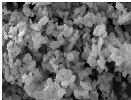
รูปที่ 4.2 ลักษณะผงอะลูมินาจากกล้องจุลทรรศน์อิเล็กตรอนแบบส่องกราด
