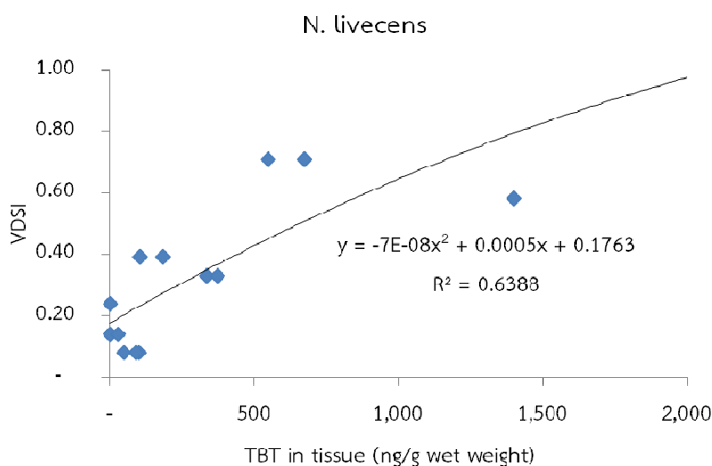
รูปที่ 13 ความสัมพันธ์ระหว่างค่าความรุนแรงในการเกิดความผิดปกติทางเพศ (ค่า VDSI) และปริมาณการสะสมของสารไตรบิวทิลทินในเนื้อเยื่อหอยทะเลชนิด N. livecens
