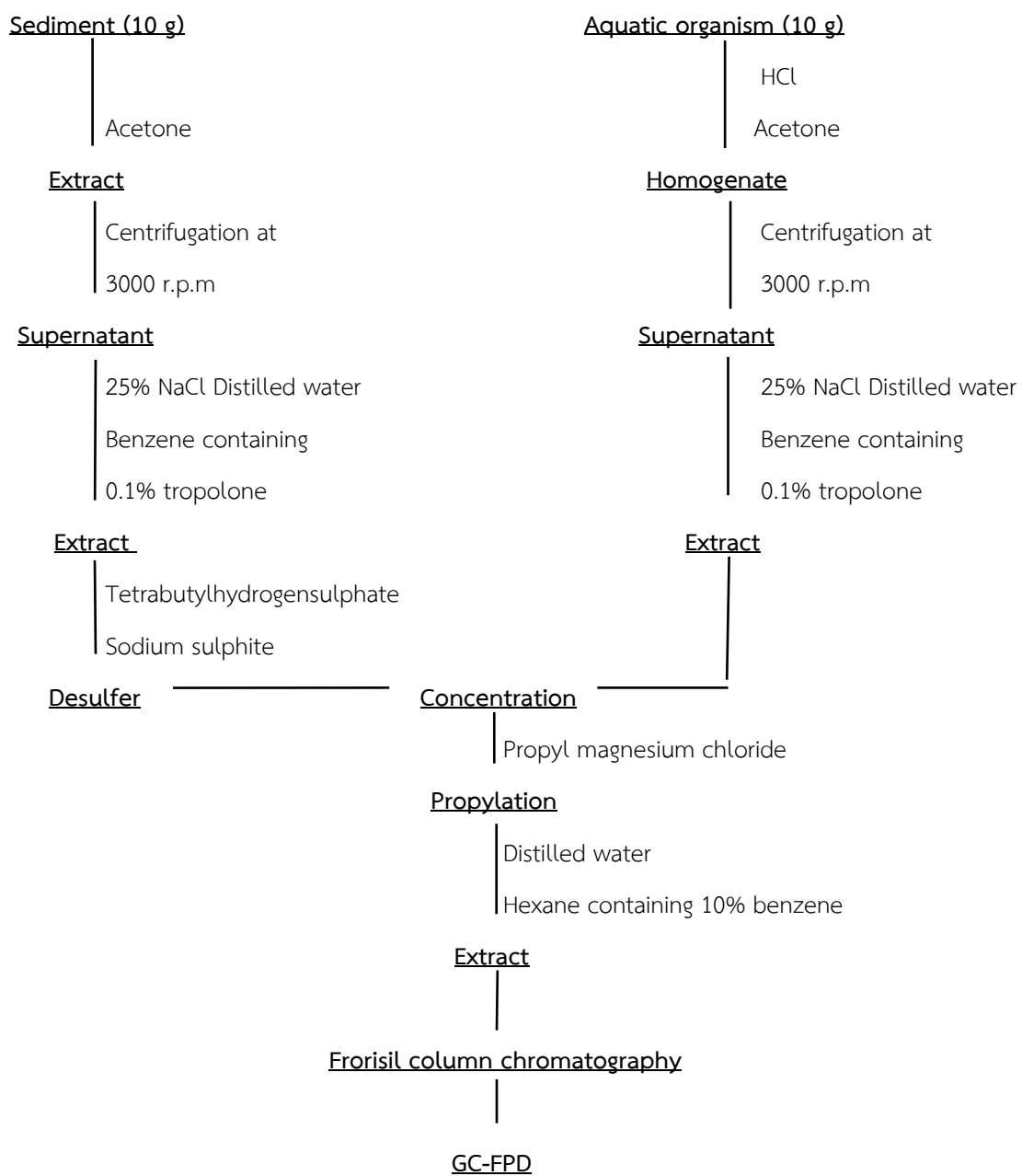
รูปที่ 4 แผนผังขั้นตอนการสกัดสารในกลุ่มออกแกโนตินในดินตะกอนและในสิ่งมีชีวิต (ปรับปรุงจาก Harino, 2003)
