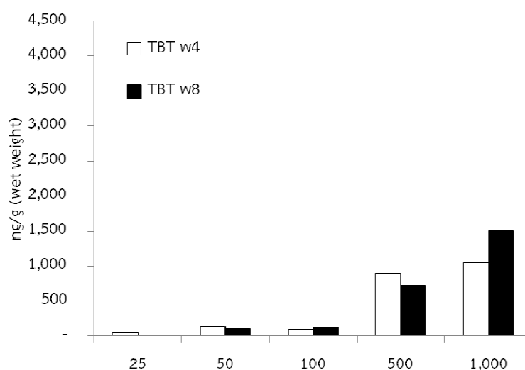
รูปที่ 17 ปริมาณการสะสมของสารไตรบิวทิลทีนในเนื้อเยื่อของหอยทะเลชนิด N. stolatus ที่ได้เลี้ยงในบ่อทดลองที่มีปริมาณการปนเปื้อนของสารไตรบิวทิลทีนคลอไรด์ที่แตกต่างกัน
