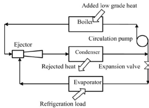
รูปที่ 2.2 ผังแสดงระบบทำความเย็นแบบอีเจกเตอร์อย่างง่าย
