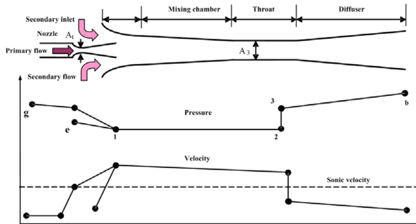
รูปที่ 2.3 ลักษณะการไหลของสารทำงานภายในอีเจกเตอร์
