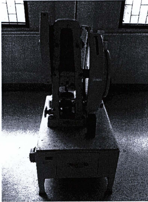
รูปที่ 2-1 เครื่องตอกยาเม็ด Single punch machine
