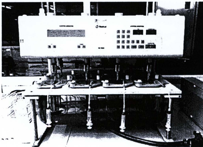
รูปที่ 2-6 เครื่องทดสอบการปลดปล่อยตัวยา
