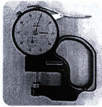
รูปที่ 2-3 เครื่องวัดความหนาเม็ดยา
