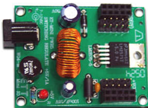
ภาพที่ ข-3 บอร์ดควบคุมแรงดัน
