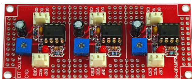
ภาพที่ ข-5 บอร์ดขยายสัญญาณเซนเซอร์
