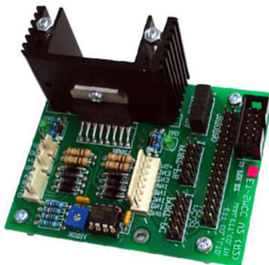
ภาพที่ ข-2 บอร์ดควบคุมมอเตอร์สองตัว
