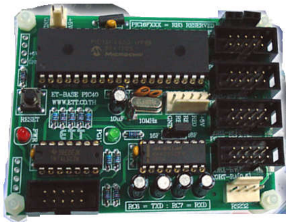
ภาพที่ ข-1 บอร์ดควบคุมหลักด้วยไมโครคอนโทรลเลอร์
