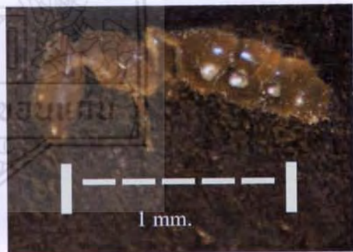
Pseudolasius spp.1
