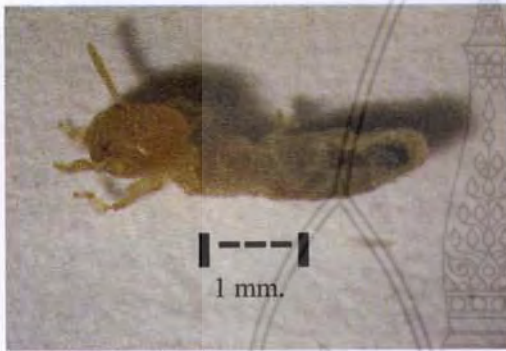
Ancistrotermes spp.
