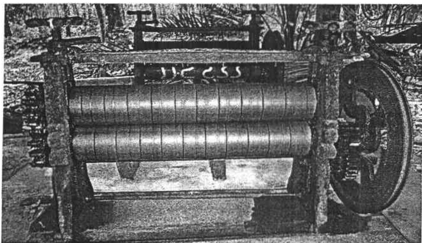
รูปที่ 3 จักรลีน เป็นอุปกรณ์ที่ทำหน้าที่ในการรีดน้ำยางที่แข็งตัว และผ่านการนวดบนแท่นนวดมาแล้ว ซึ่งในการรีดแผ่นยางจะต้องรีดจนกระทั่งแผ่นยางมีความหนาประมาณ 2-3 มิลลิเมตร
