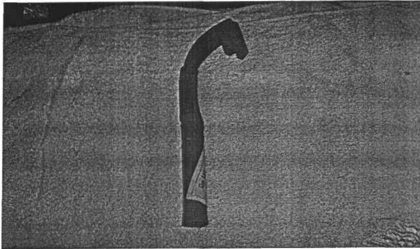
รูปที่ 1 มีดกรีดยาง เป็นอุปกรณ์ที่มีความสำคัญมากในการประกอบอาชีพกรีดยาง ทั้งนี้เนื่องจาก มีดกรีดยาง จะเป็นอุปกรณ์ที่ใช้สำหรับเฉือนเปลือกยาง เพื่อตัดผ่านท่อน้ำยาง และทำให้น้ำยางจะไหลออกมา
