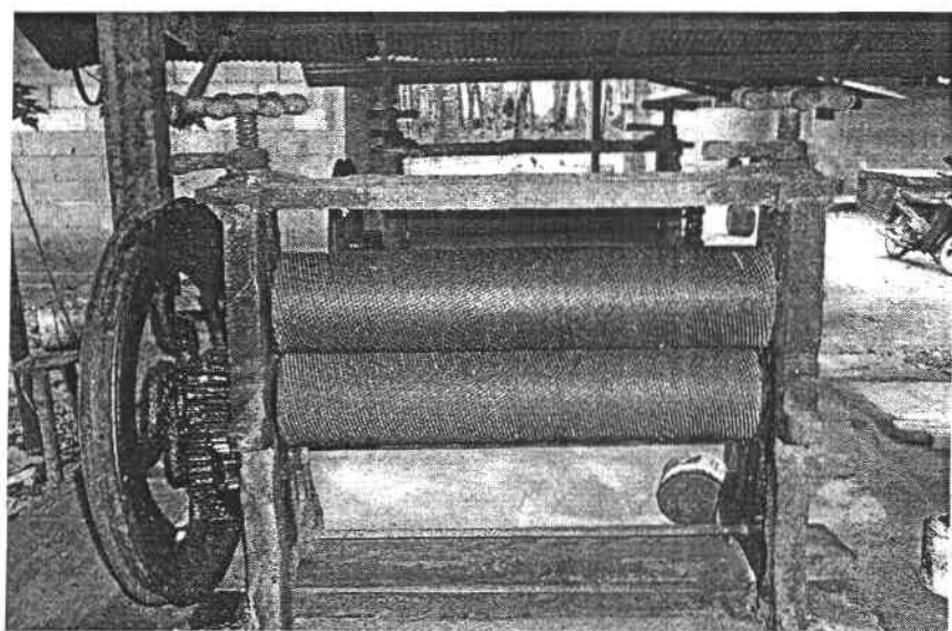
รูปที่ 4 จักรดอก ทำหน้าที่ในการรีดแผ่นยางพารา หลังจากยางพาราผ่านการรีดด้วยจักรลีนมาแล้ว
