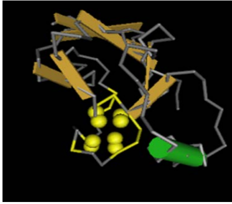
รูปที่ 10 : โครงสร้างสามมิติของ Ferredoxin
