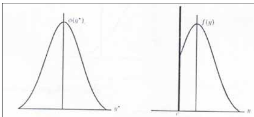
ภาพที่ 1 ฟังก์ชันความหนาแน่นของตัวแปรสุ่มที่มีการแจกแจงแบบปกติของ y^* และตัวแปรสุ่ม y ที่ถูกตัด
