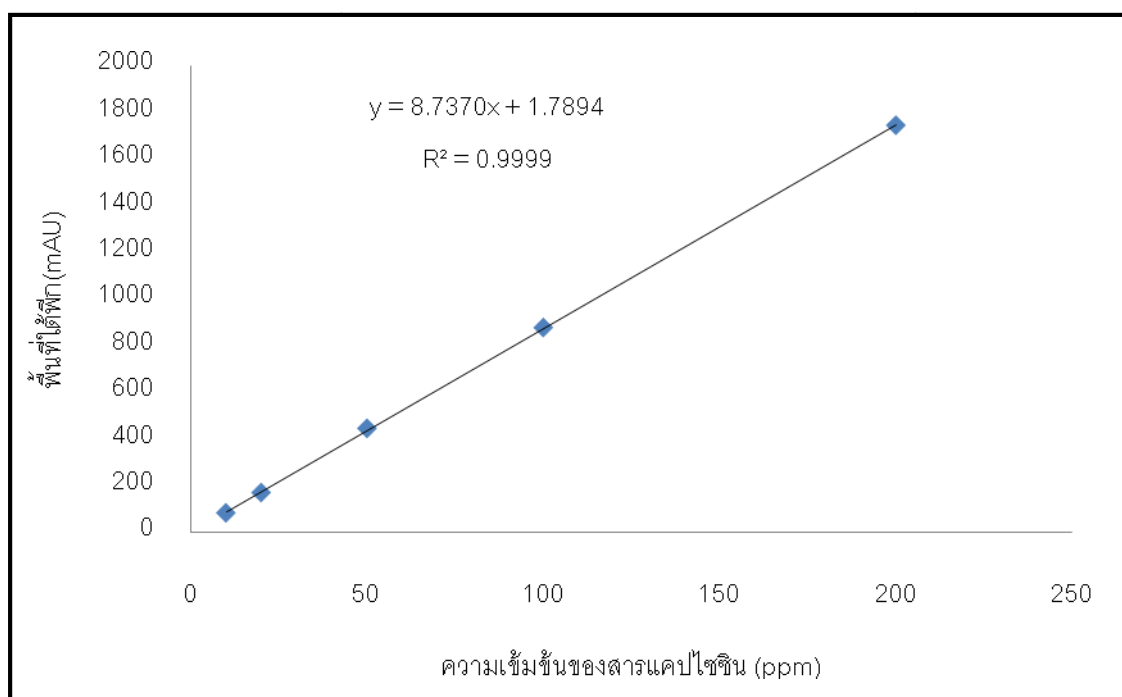
รูปที่ ๒ มาตรฐานความสัมพันธ์ระหว่างพื้นที่ใต้ peak และความเข้มข้นของสาร capsaicin
