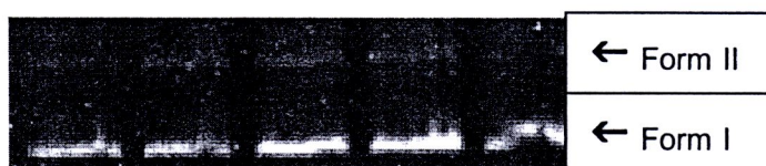
รูปที่ 4.9 แสดงแผนภาพอิเล็กโทรโฟรีซิสของ plasmid DNA pUC18 ที่ความเข้มข้นต่างๆ ของสารสกัดแม็ก: (A) control; (B) 1 \mu\text{g/ml} ; (C) 5 \mu\text{g/ml} ; (D) 25 \mu\text{g/ml} ; และ (E) 50 \mu\text{g/ml}
