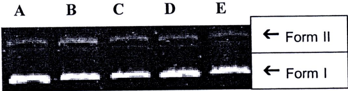
รูปที่ 4.5 แสดงแผนภาพอิเล็กโทรโฟรีซิสของ plasmid DNA pUC18 ที่ความเข้มข้นต่างๆ ของสารมาตรฐาน quercetin (A) control; (B) 1 µg/ml; (C) 5 µg/ml; (D) 25 µg/ml; และ (E) 50 µg/ml
