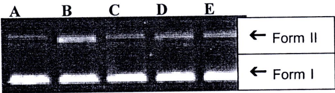
รูปที่ 4.4 แสดงแผนภาพอิเล็กโทรโฟรีซิสของ plasmid DNA pUC18 ที่ความเข้มข้นต่างๆ ของสารสกัดสมอเทศ : (A) control; (B) 1 µg/ml; (C) 5 µg/ml; (D) 25 µg/ml; และ (E) 50 µg/ml
