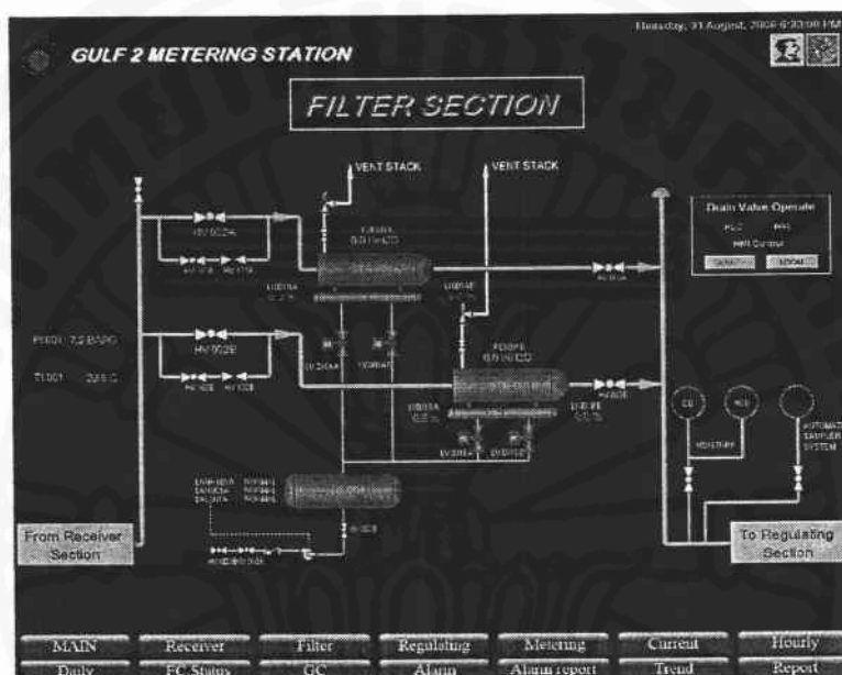
ภาพที่ ก.6 ระบบท่อนำส่งก๊าซ ของ ปตท
