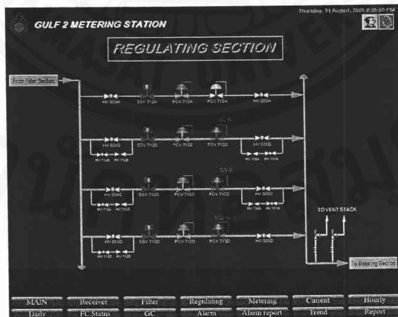
ภาพที่ ก.13 การควบคุมการทำงาน ในท่อนำส่งก๊าซ ของปตท
