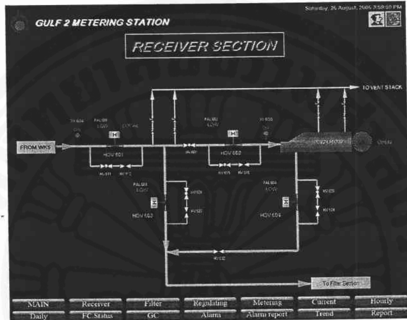
ภาพที่ ก.12 การรับส่ง ก๊าซ ในท่อนำส่งก๊าซ ของปตท
