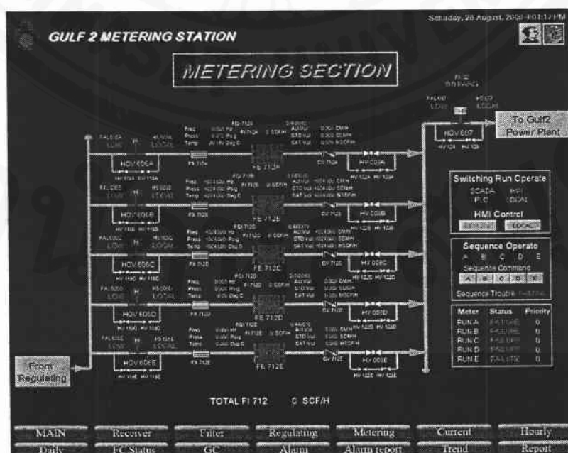
ภาพที่ ก.11 การทำงานของมิเตอร์ในท่อนำส่งก๊าซ ของปตท
