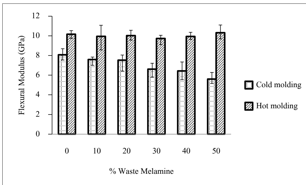
รูปที่ 4.2 กราฟแสดงความสัมพันธ์ระหว่างค่ามอดูลัสและร้อยละปริมาณเศษเมลามีน
