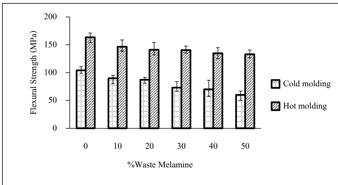
รูปที่ 4.1 กราฟแสดงความสัมพันธ์ระหว่างความแข็งแรงดัดและร้อยละปริมาณเศษเมลามีน
