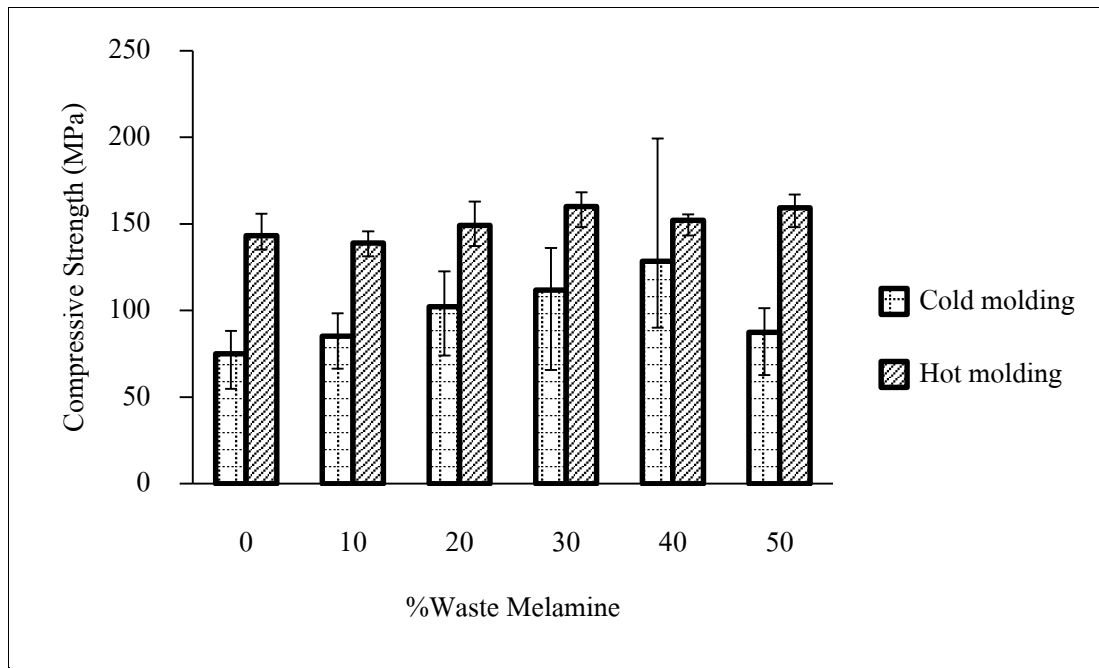
รูปที่ 4.4 กราฟแสดงความสัมพันธ์ระหว่างความแข็งแรงอัดและร้อยละปริมาณเศษเมลามีน
