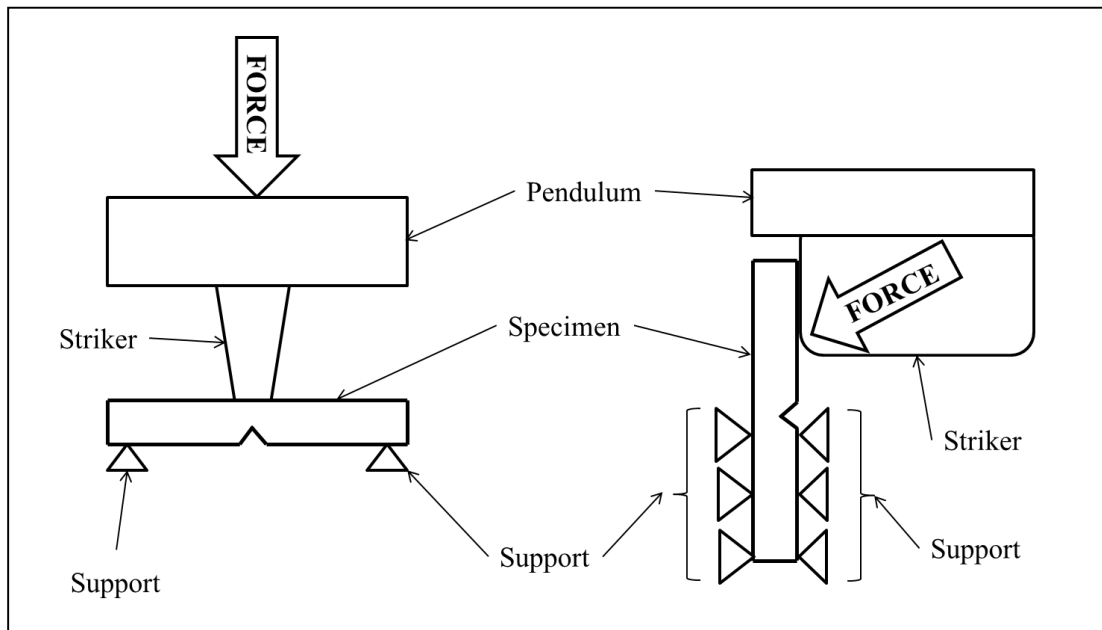
รูปที่ 2.8 ขั้นตอนทดสอบการกระแทกแบบชาร์ปีและไอซอด
