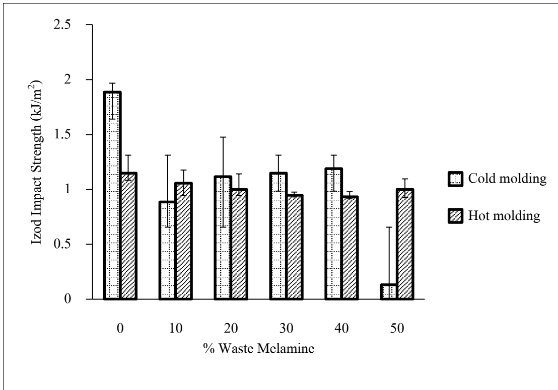
รูปที่ 4.3 กราฟแสดงความสัมพันธ์ระหว่างความแข็งแรงกระแทกและร้อยละปริมาณเศษเมลามีน
