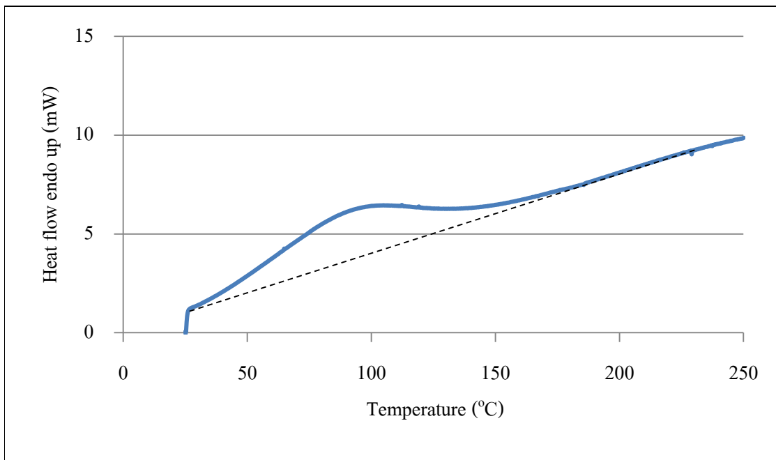
รูปที่ 4.10 กราฟ DSC ของวัสดุที่ขึ้นรูปด้วยการอัดเย็น
