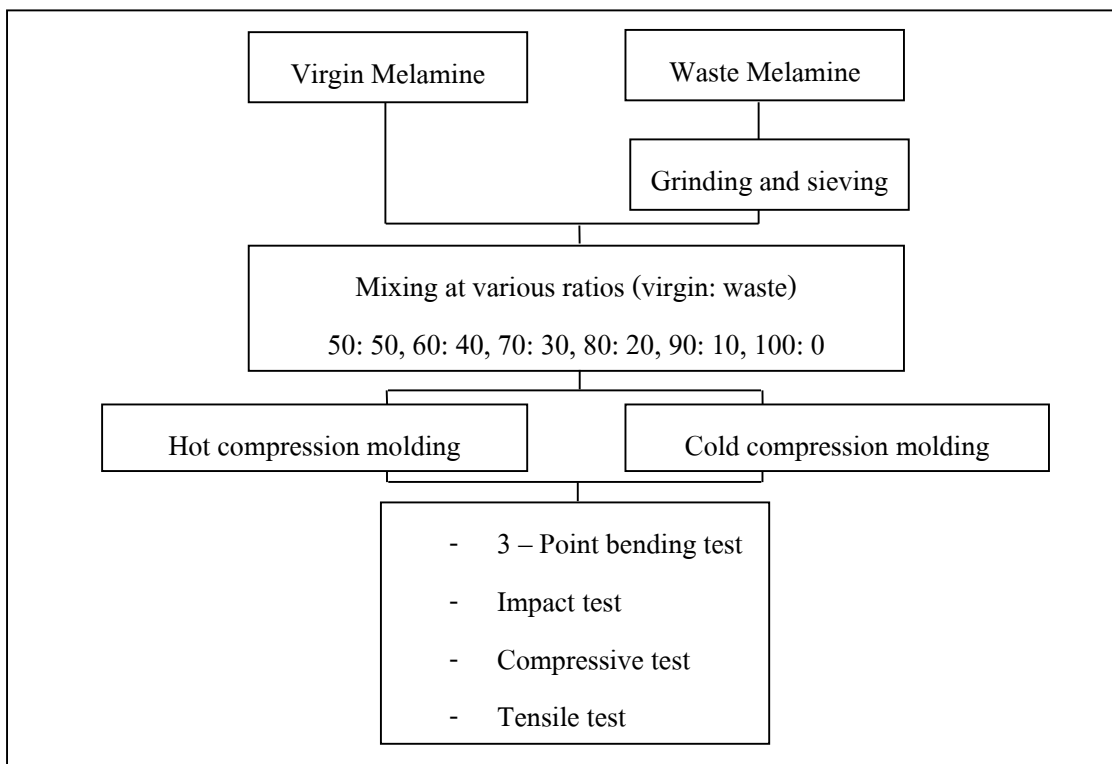
รูปที่ 3.1 แผนผังแสดงขั้นตอนการดำเนินงานโดยสังเขป
