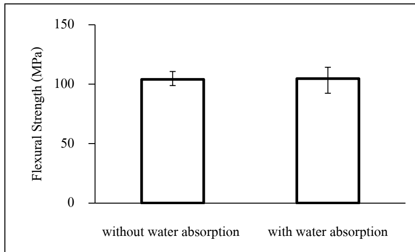
รูปที่ 4.5 กราฟแสดงความสัมพันธ์ระหว่างความแข็งแรงดัดของชิ้นทดสอบการดูดซึมน้ำ
