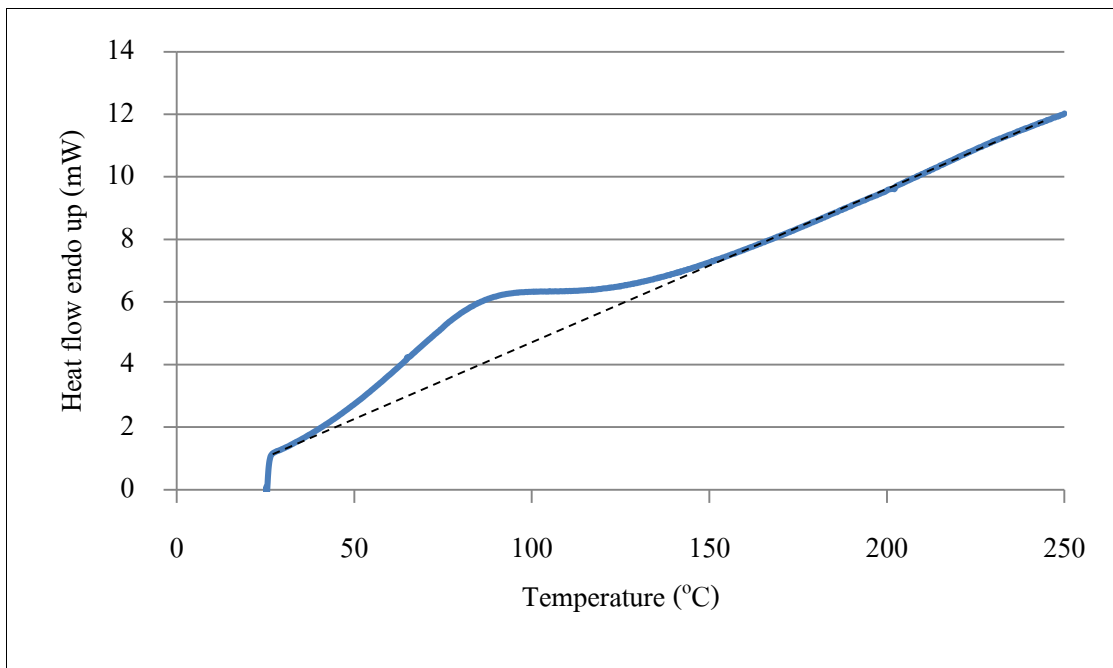
รูปที่ 4.9 กราฟ DSC ของวัสดุที่ขึ้นรูปด้วยการอัดรีด
