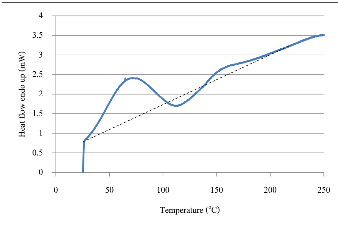
รูปที่ 4.8 กราฟ DSC ของสารประกอบเมลามีน (Melamine Compound)
