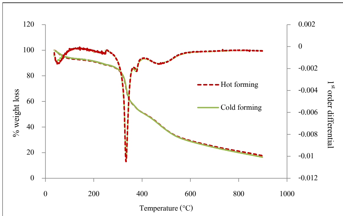
รูปที่ 4.7 กราฟ TGA ของเมลามีนเมื่อเปลี่ยนวิธีการขึ้นรูปแบบอัดร้อนและอัดเย็น
