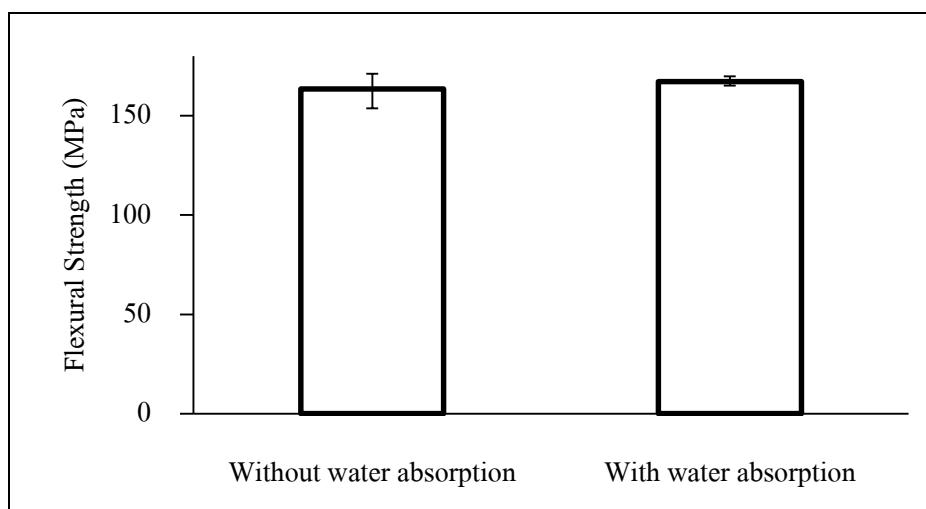
รูปที่ 4.6 กราฟแสดงความสัมพันธ์ระหว่างความแข็งแรงดัดของชิ้นทดสอบการดูดซึมน้ำ
