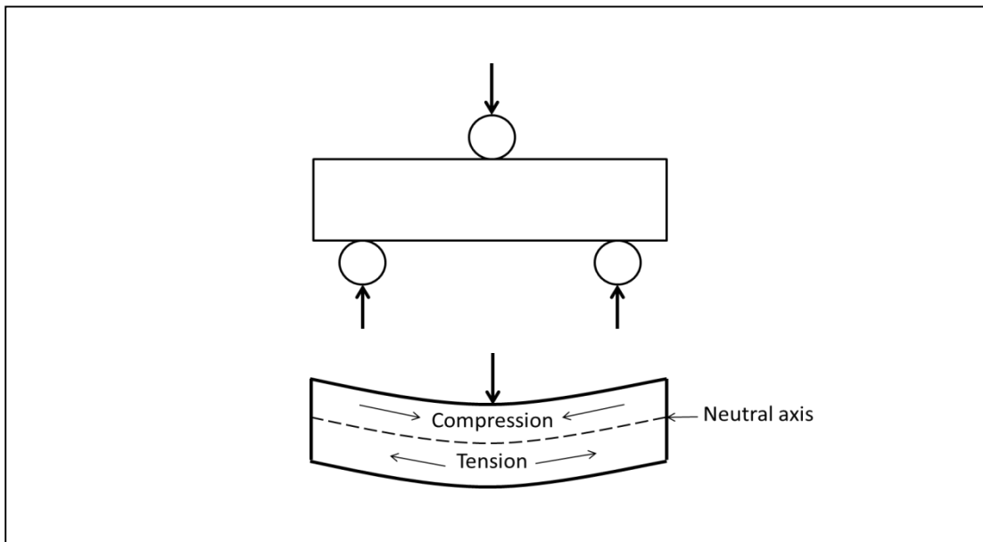
รูปที่ 2.3 ลักษณะการทดสอบแรงดัดงอแบบจุดสามจุด
