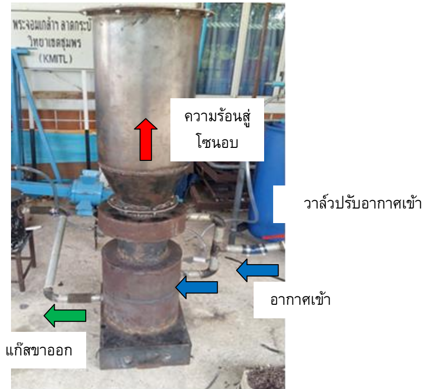
รูปที่ ค-2 ตำแหน่งการเดินทางของแก๊สชีวมวล
