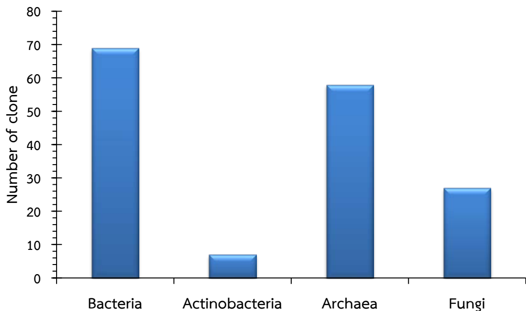
ภาพที่ 4-1 จำนวนโคลนของจุลินทรีย์กลุ่มแบคทีเรียทั่วไป แอคทีโนแบคทีเรียและอาร์เคียที่ปรากฏในห้องสมุดยีน 16S rRNA ของจุลินทรีย์แต่ละกลุ่ม และจำนวนโคลนของจุลินทรีย์กลุ่มรา (ราสายและยีสต์) ที่ปรากฏในห้องสมุด ITS จากเมตาจีโนมของดินนาเกลือในจังหวัดฉะเชิงเทรา
