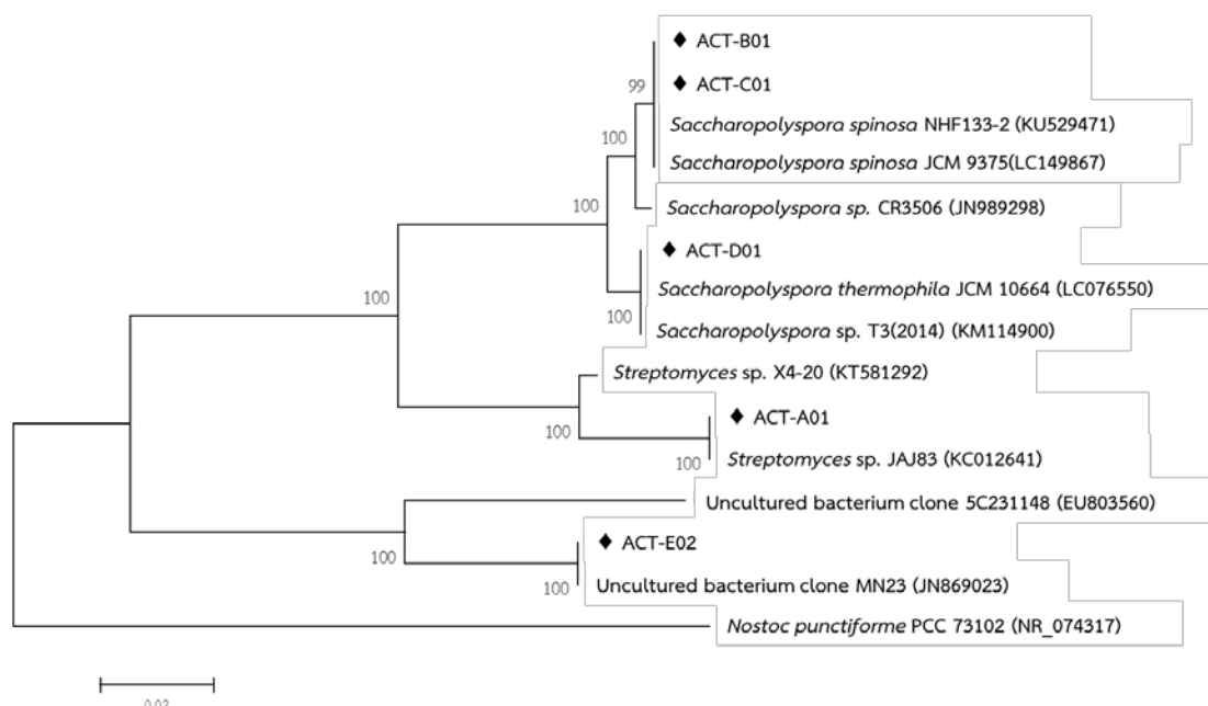
ภาพที่ 4-4 แผนภูมิสายสัมพันธ์เชิงวิวัฒนาการของแอกทีโนแบคทีเรียที่พบในเมตาจีโนมของดินนาเกลือ สร้างขึ้นด้วยวิธี Neighbor-Joining บนโปรแกรม MEGA 6 โดยอาศัยข้อมูลลำดับนิวคลีโอไทด์ของยีน 16S rRNA และใช้ p-distance ในการคำนวณระยะห่างทางวิวัฒนาการ ซึ่งปรากฏเป็นความยาวกิ่งของแอกทีโนแบคทีเรียแต่ละแทกซอน ทดสอบความเชื่อมั่นของแผนภูมิโดยวิธี Bootstrapping จำนวน 1,000 ซ้ำ ลำดับนิวคลีโอไทด์ของยีน 16S rRNA จำนวน 1,341 ตำแหน่ง ของข้อมูลลำดับนิวคลีโอไทด์ทั้งหมด 15 ข้อมูล ถูกนำมาใช้ในการวิเคราะห์และสร้างสายสัมพันธ์เชิงวิวัฒนาการ โดยมี Nostoc punctiforme (NR_074317) เป็นแทกซอนนอกกลุ่ม
