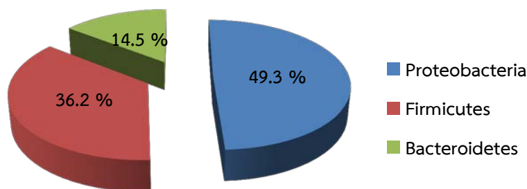
ภาพที่ 4-2 ความถี่ของการพบแบคทีเรียไฟลัมต่างๆ จากโคลนที่ปรากฏในห้องสมุดยีน 16S rRNA ซึ่งได้จากเมตาจีโนมของดินนาเกลือในพื้นที่จังหวัดฉะเชิงเทรา
