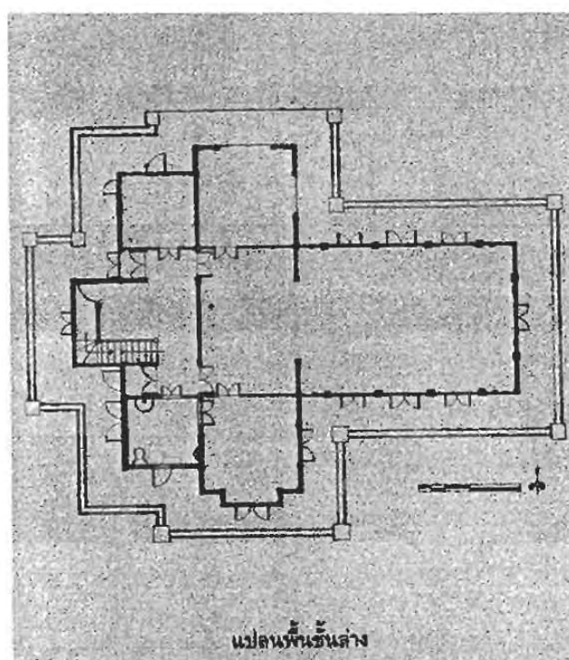
แผนผังที่ 2 ผังพื้นชั้นล่าง พระตำหนักมารีราชรัตบัลลังก์
