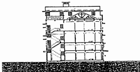
แผนผังที่ 75 รูปตัด C - C อาคาร 3 กลุ่มอาคารริมถนนราชดำเนินกลาง
