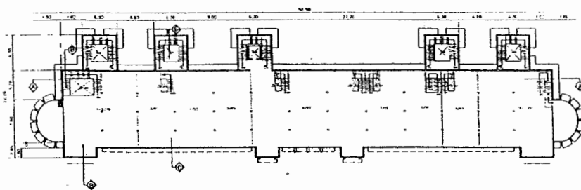
แผนผังที่ 184 ผังอาคารชั้น 2 อาคาร 13 กลุ่มอาคารริมถนนราชดำเนินกลาง
