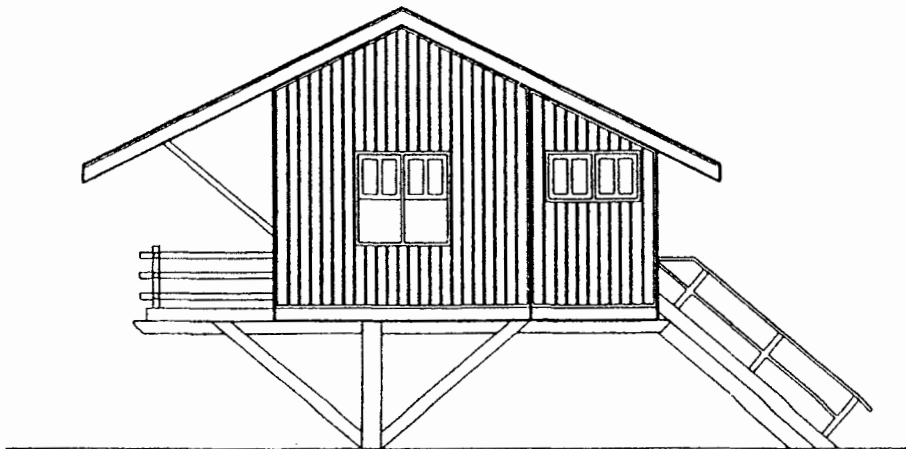
แผนผังที่ 274 รูปด้าน 2 บ้านสองเสา
