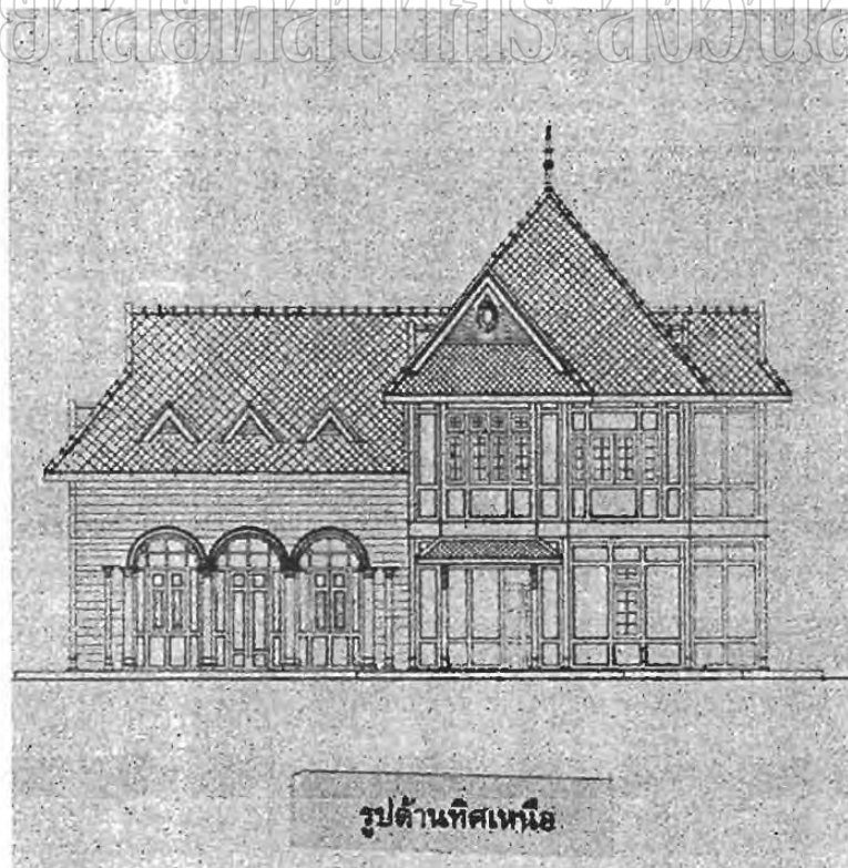
แผนผังที่ 5 รูปด้านทิศเหนือ พระตำหนักมหาราชรัศมีดั่งกั
