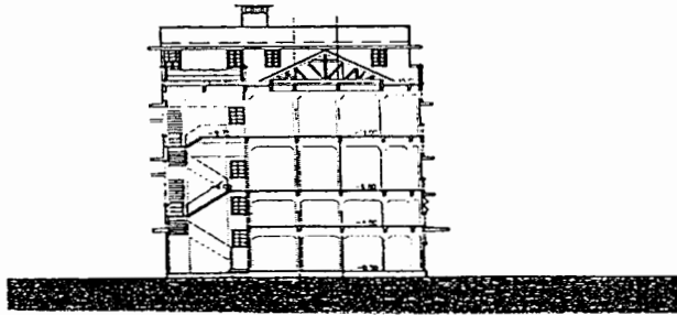
แผนผังที่ 136 รูปตัด C - C อาคาร 8 กลุ่มอาคารริมถนนราชดำเนินกลาง
