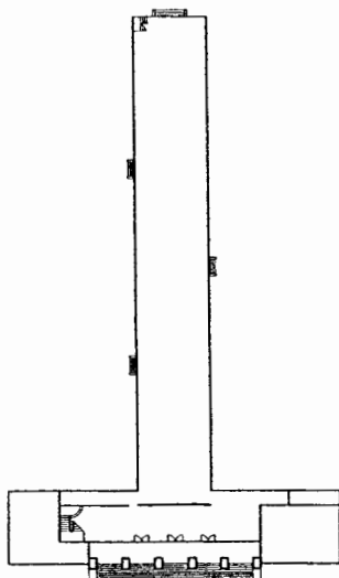
แผนผังที่ 243 ผังอาคารชั้นล่าง อาคารศาลากลางจังหวัดพระนครศรีอยุธยา(หลังเก่า)
