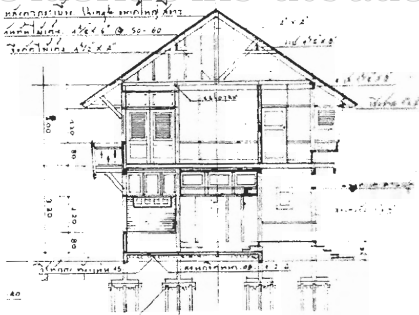
แผนผังที่ 271 รูปตัดอาคาร
