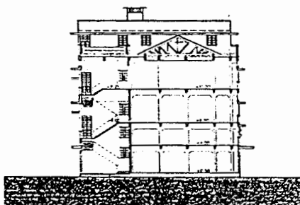
แผนผังที่ 51 รูปตัด C - C อาคาร 1 กลุ่มอาคารริมถนนราชดำเนินกลาง
