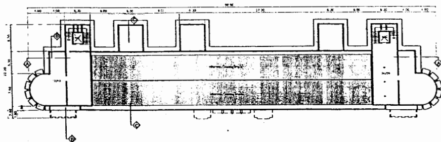
แผนผังที่ 166 ผังอาคารชั้น 4 อาคาร 11 กลุ่มอาคารริมถนนราชดำเนินกลาง
