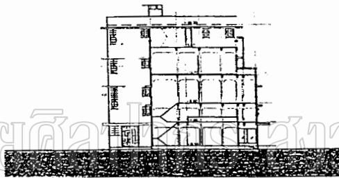
แผนผังที่ 74 รูปตัด B - B อาคาร 3 กลุ่มอาคารริมถนนราชดำเนินกลาง
