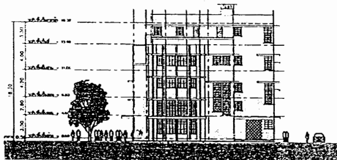
แผนผังที่ 111 รูปด้าน 3 อาคาร 6 กลุ่มอาคารริมถนนราชดำเนินกลาง
