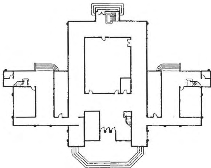
แผนผังที่ 225 ผังอาคารชั้นล่าง ศาลแขวงสงขลา
