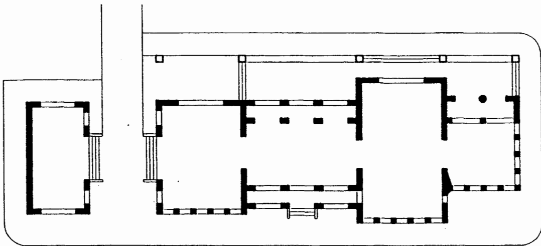
แผนผังที่ 12 ผังอาคารของพระตำหนักสมเด็จพระเจ้าฟ้ากรมหลวงสงขลานครินทร์
