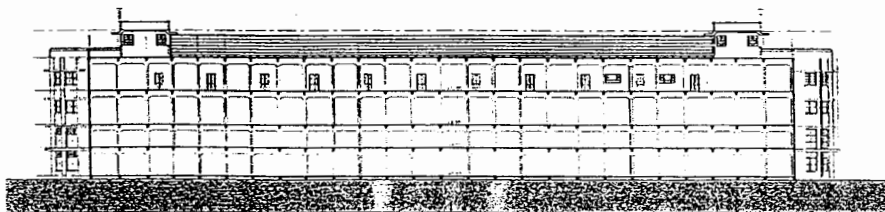
แผนผังที่ 49 รูปตัด A - A อาคาร 1 กลุ่มอาคารริมถนนราชดำเนินกลาง
