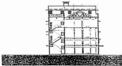
แผนผังที่ 190 รูปตัด C - C อาคาร 13 กลุ่มอาคารริมถนนราชดำเนินกลาง
