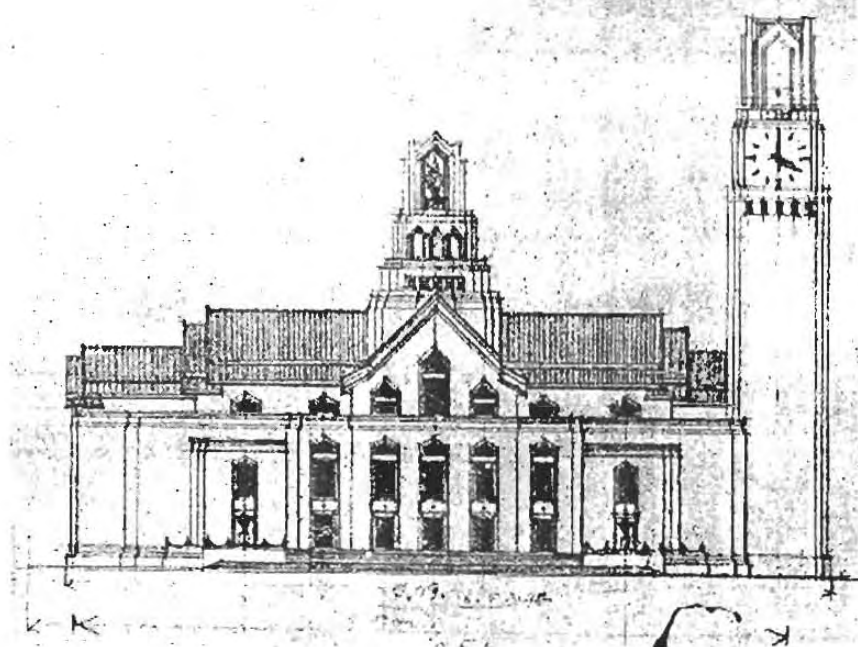
แผนผังที่ 16 แบบร่างรูปด้านศาตศาตศบาลนครกรุงเทพ ด้านหน้า
