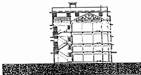
แผนผังที่ 88 รูปตัด B - B อาคาร 4 กลุ่มอาคารริมถนนราชดำเนินกลาง
