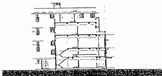
แผนผังที่ 121 รูปตัด B - B อาคาร 7 กลุ่มอาคารริมถนนราชดำเนินกลาง
