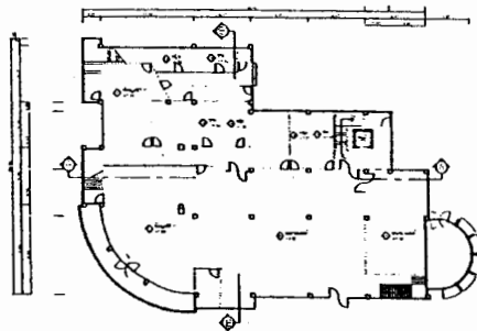
แผนผังที่ 150 ผังอาคารชั้นล่าง อาคาร 10 กลุ่มอาคารริมถนนราชดำเนินกลาง
