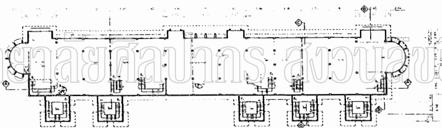
แผนผังที่ 107 ผังอาคารชั้นลอย อาคาร 6 กลุ่มอาคารริมถนนราชดำเนินกลาง
