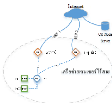
ภาพที่ 1: เครือข่ายเซนเซอร์ไร้สายแบบ 2 เกตเวย์
