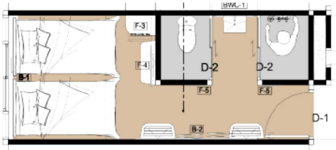
ภาพที่ 5.4 รูปแบบการออกแบบร่างของตกแต่งภายในห้องพัก โครงการ ดิ เอ็กซ์ ทริม
