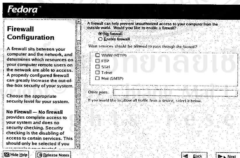
จากรูปที่ ก.13 การกำหนดไฟร์วอลล์
