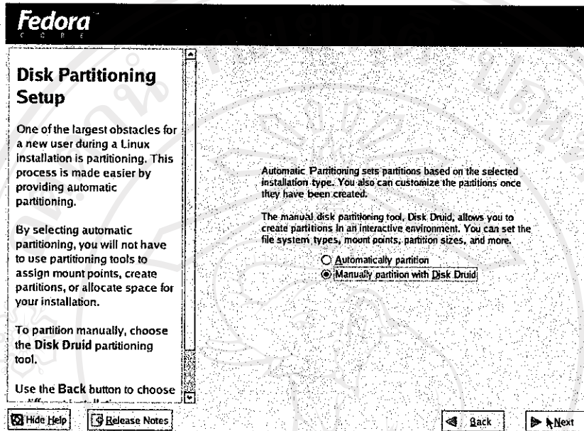
รูปที่ ก.10 การแบ่งพาร์ติชัน
