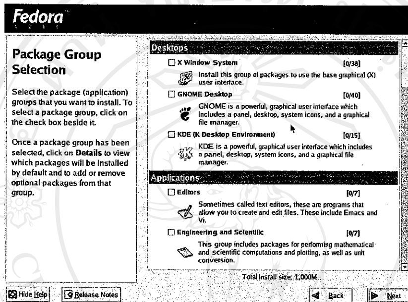
รูปที่ ก.18 เลือกโปรแกรมสำหรับการติดตั้ง
