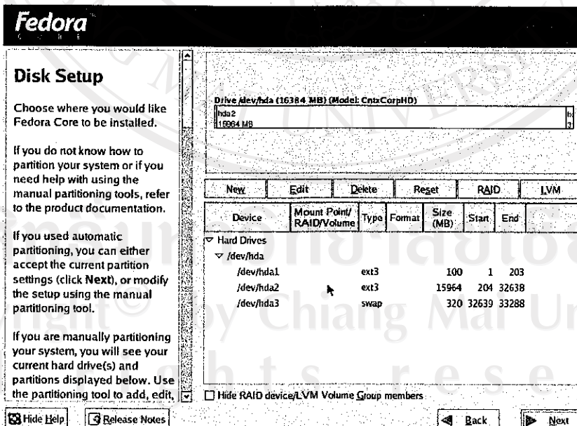
รูปที่ ก.11 การจัดการพาร์ติชัน
