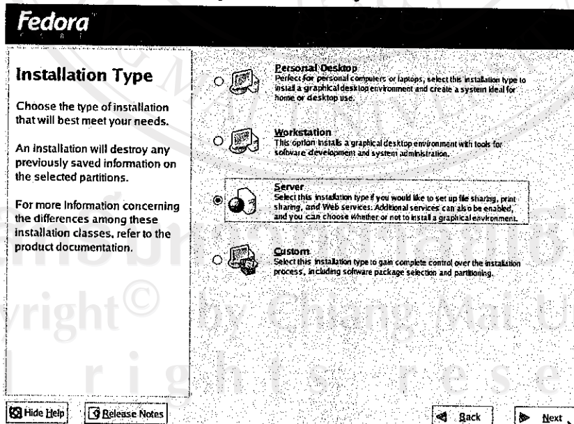
รูปที่ ก.9 เลือกประเภทการติดตั้ง โปรแกรม ในที่นี้เลือกการลงแบบเซิร์ฟเวอร์
