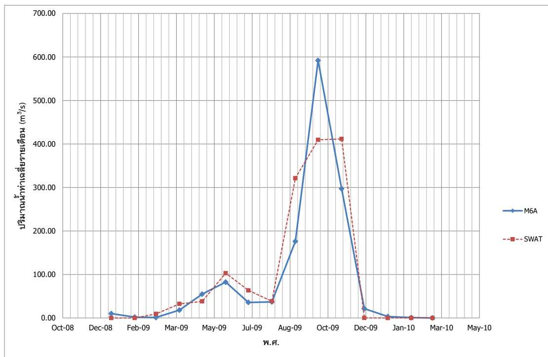
ภาพที่ 4.1-6 การตรวจพิสูจน์ค่าปริมาณน้ำท่าเฉลี่ยรายเดือน ณ สถานีวัดน้ำท่า M.6A
