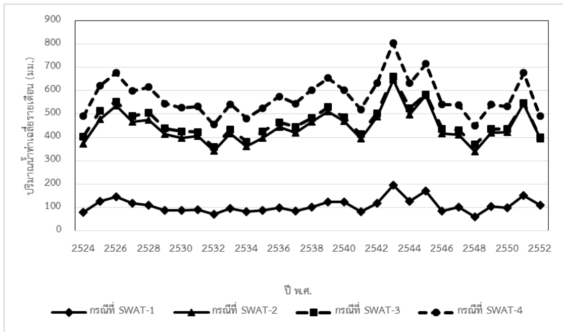
ภาพที่ 4.1-7 ปริมาณน้ำท่าเฉลี่ยรายปีสำหรับทั้ง 4 กรณีส
