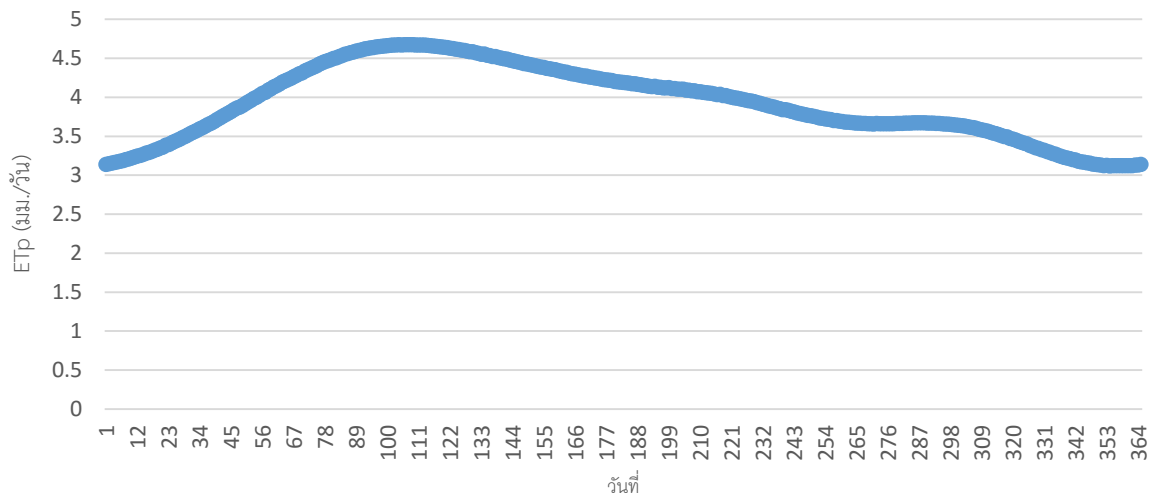
รูปที่ 3.4 ผลการคำนวณค่า ETp รายวันตลอดปีจากแบบจำลอง ANN ของพื้นที่ฟาร์มม.เทคโนโลยีสุรนารี
