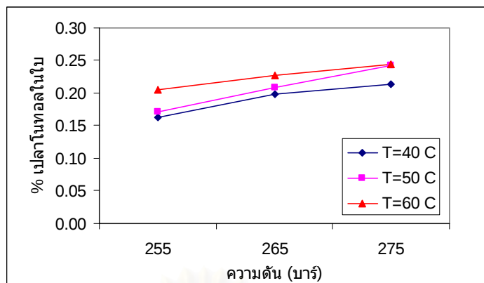
รูปที่ 4.6 ผลของความดันต่อปริมาณเปลาโนทอลในใบ ที่สกัดได้ที่อัตราการไหลของ คาร์บอนไดออกไซด์ = 3 กรัม/นาที
