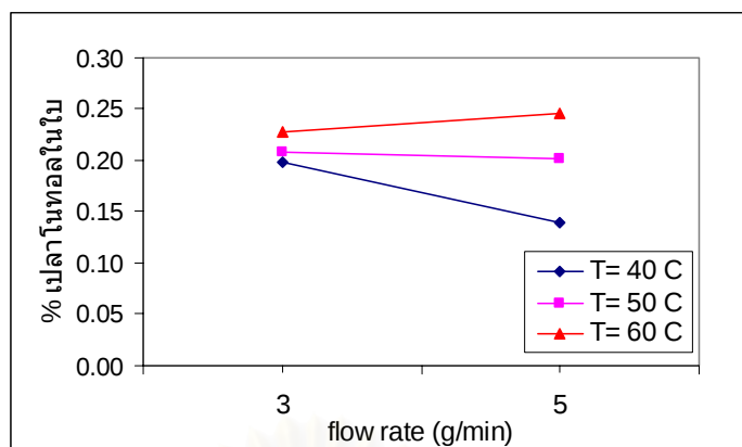
รูปที่ 4.11 ผลของอัตราการไหลของคาร์บอนไดออกไซด์ต่อปริมาณเปลาโนทอลในใบ ทั้งหมดที่สกัดได้ ที่ความดัน 265 บาร์
