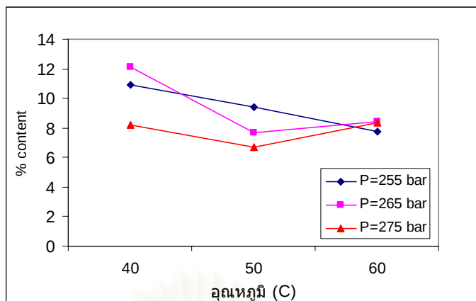
รูปที่ 4.4 ผลของอุณหภูมิต่อปริมาณของเปลาโนทอลในส่วนสกัด ที่สกัดได้ ที่อัตราการไหลของคาร์บอนไดออกไซด์ = 3 กรัม/นาที
