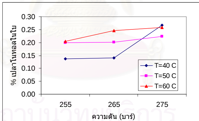
รูปที่ 4.7 ผลของความดันต่อปริมาณเปลาโนทอลในใบ ที่สกัดได้ที่อัตราการไหลของ คาร์บอนไดออกไซด์ = 5 กรัม/นาที
