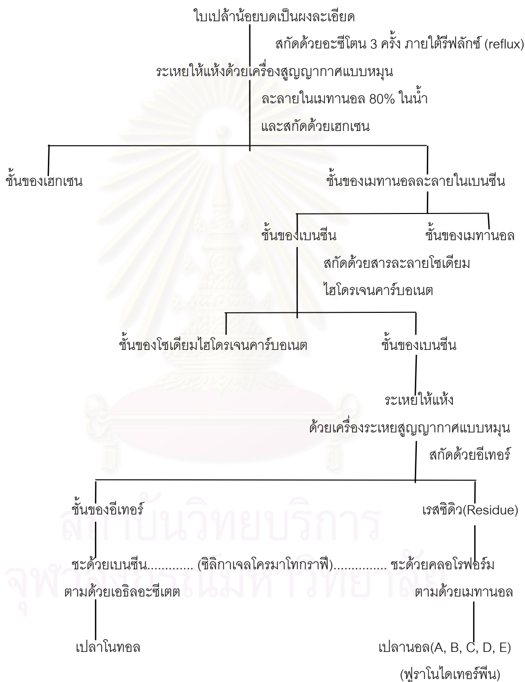
รูปที่ 2.19 แผนภาพขั้นตอนการสกัดเปลาโนทอลของบริษัทซังเกียว (24)
