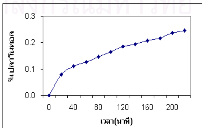
รูปที่ ค.15 เปอร์เซนต์เปลาโนทอลในใบ ได้จากภาวะการทดลองที่ 15
