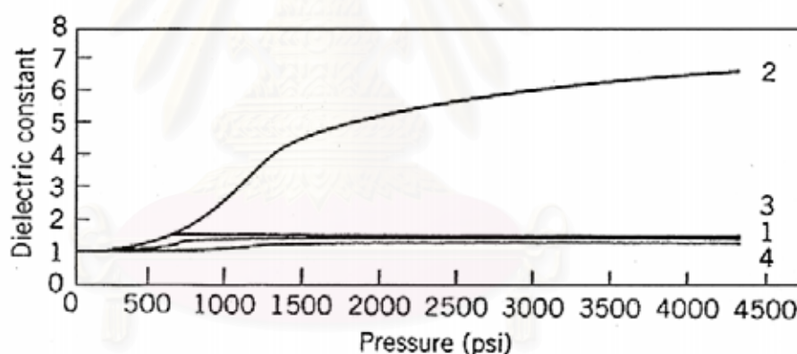
รูปที่ 2.25 ผลของความดันที่มีต่อสภาพขั้วของ อีเทน (เส้น 4), โพรเพน (เส้น 3), ฟลูออโรฟอร์ม(เส้น 2), และซัลเฟอร์เฮกซะฟลูออไรด์ (เส้น 1) ที่อุณหภูมิ 50 องศาเซลเซียส (23)
