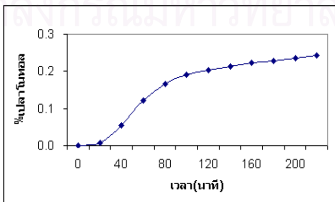
รูปที่ ค.8 เปอร์เซนต์เปลาโนทอลในใบ จากภาวะการทดลองที่ 8
