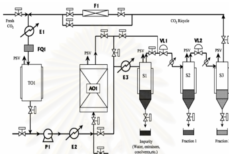
รูปที่ 3.2 แผนผังการสกัดด้วยคาร์บอนไดออกไซด์ภาวะเหนือวิกฤต (pilot scale)
