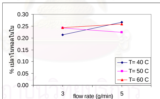
รูปที่ 4.12 ผลของอัตราการไหลของคาร์บอนไดออกไซด์ต่อปริมาณเปลาโนทอลในใบ ทั้งหมดที่สกัดได้ ที่ความดัน 275 บาร์
