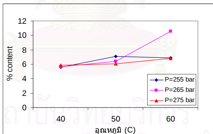
รูปที่ 4.5 ผลของอุณหภูมิต่อปริมาณของเปลาโนทอลในส่วนสกัด ที่สกัดได้ ที่อัตราการไหลของคาร์บอนไดออกไซด์ = 5 กรัม/นาที
