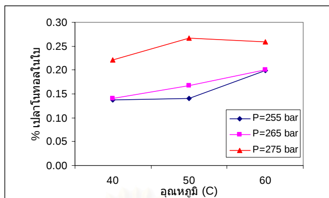
รูปที่ 4.3 ผลของอุณหภูมิต่อปริมาณเปลาโนทอลในโบ ที่สกัดได้ ที่อัตราการไหลของคาร์บอนไดออกไซด์ = 5 กรัม/นาที่
