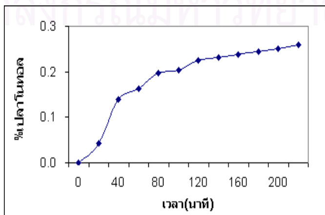
รูปที่ ค.18 เปอร์เซนต์เปลาโนทอลในใบ ได้จากภาวะการทดลองที่ 18
