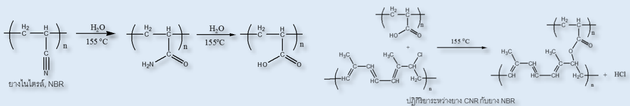
รูปที่ 2 ปฏิกริยาระหว่างยางธรรมชาติคลอรีนกับยางไนไตรล์
