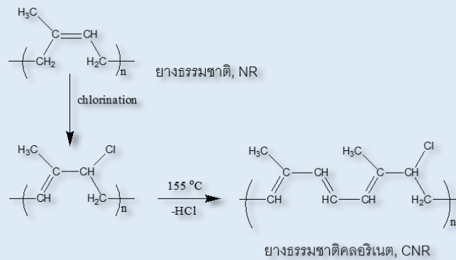
รูปที่ 1 ปฏิกริยาการสังเคราะห์ยางธรรมชาติคลอรีน
