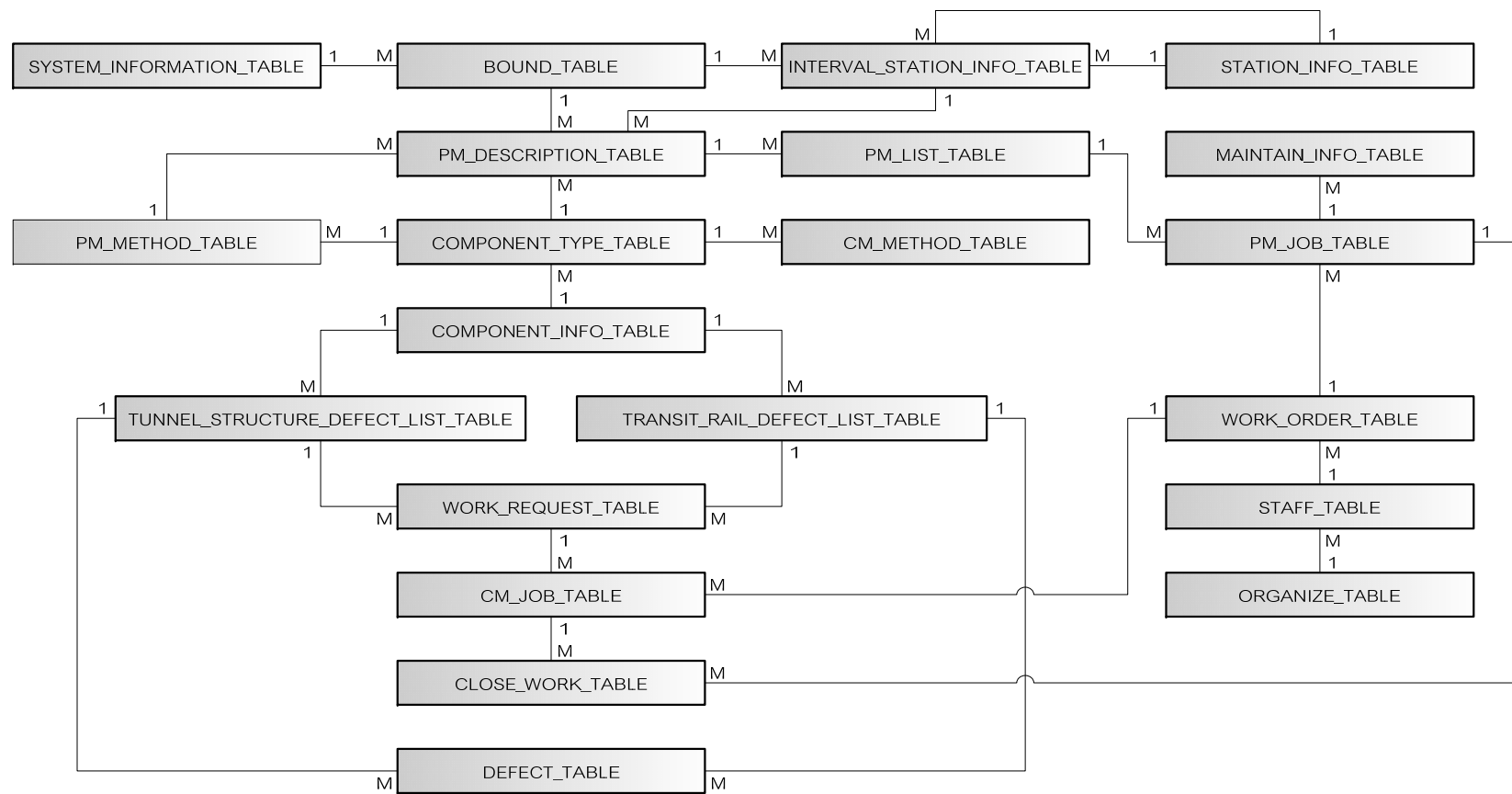
รูปที่ ก.1 แบบจำลองความสัมพันธ์ของฐานข้อมูลระบบบริหารจัดการงานบำรุงรักษาอุโมงค์รถไฟฟ้าใต้ดิน หมายเหตุ: แสดงเฉพาะตารางข้อมูลหลักเท่านั้น
