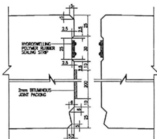
รูปที่ 4.4 แผ่นยางกันซึมและแผ่นยางบิทูมินัสบริเวณรอยต่อระหว่างชิ้นส่วนและวงแหวนอุโมงค์ (กิจการร่วมค้า ไอโอเอ็น, 2547)
