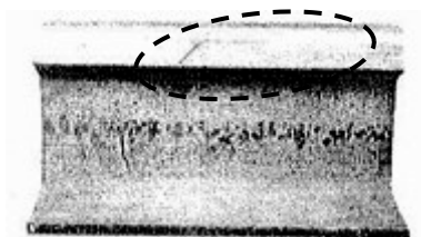
รูปที่ 4.22 รอยแตกแนวยาวของหัวราง (กิจการร่วมค้า ซีเคเอสแอล, 2545)
