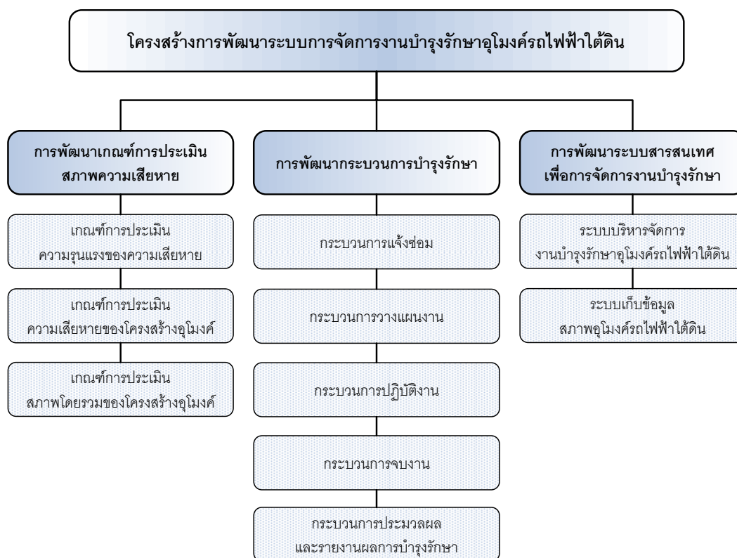
รูปที่ 5.1 โครงสร้างการพัฒนาระบบการจัดการงานการบำรุงรักษาอุโมงค์รถไฟใต้ดิน
