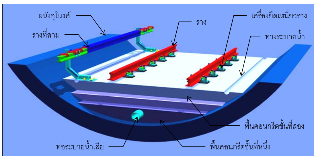
รูปที่ 4.6 ภาพตัดอุโมงค์รถไฟไฟฟ้าใต้ดินในทางตรง (กิจการร่วมค้า ซีเคเอสแอล, 2545)
