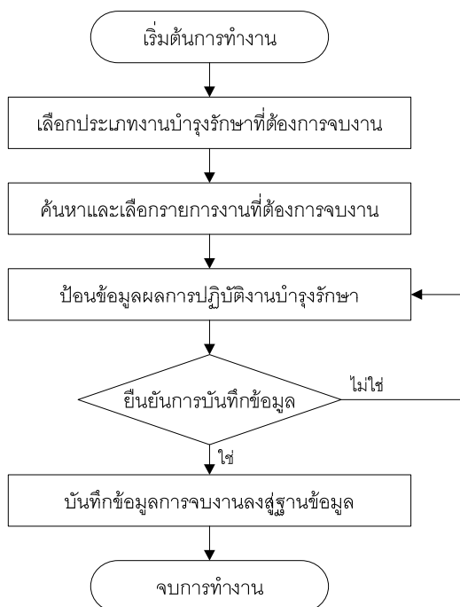
รูปที่ 6.22 การทำงานของมอดูลการจบงาน
