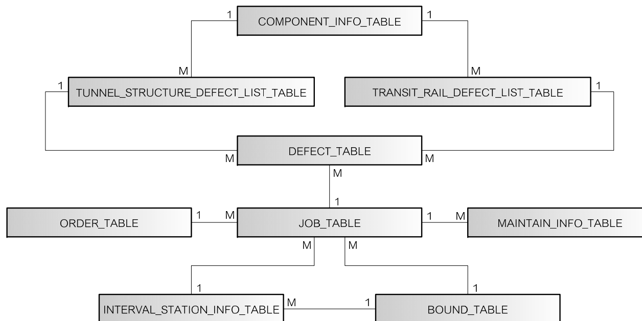
รูปที่ ก.2 แบบจำลองความสัมพันธ์ของฐานข้อมูลระบบเก็บข้อมูลสภาพภูมิวงจรไฟฟ้าใต้ดิน หมายเหตุ: แสดงเฉพาะตารางข้อมูลหลักเท่านั้น
