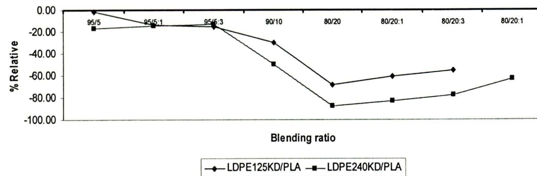
(D) Relative elongation at break
