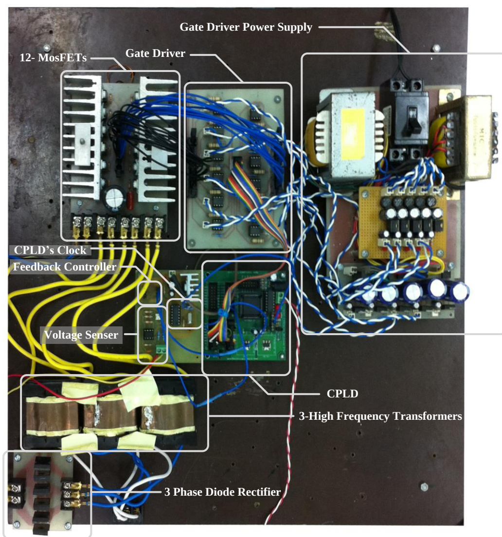
รูปที่ ก.1 ภาพจริงของวงจรแปลงผันไฟฟ้ากระแสตรงชนิดวีซิกส์ ที่มีอัตราส่วนการแปลงผันสูงโดยใช้ซีพียูแอลดี
