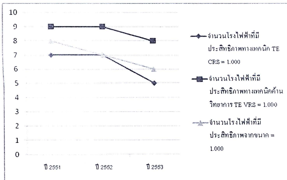
รูป 6-1 กราฟแสดงแนวโน้มจำนวนโรงไฟฟ้าที่มีประสิทธิภาพ ระหว่างปี 2551-2553
