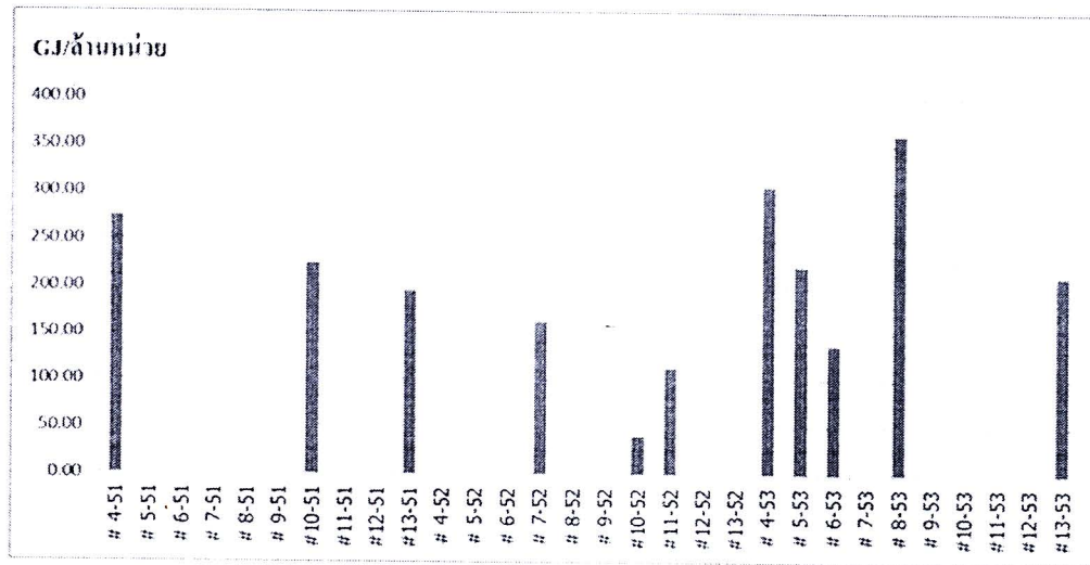
รูป 6-8 ส่วนเกินความร้อนจากเชื้อเพลิงทั้งหมด ปี 2551-53 (CCR Model)
