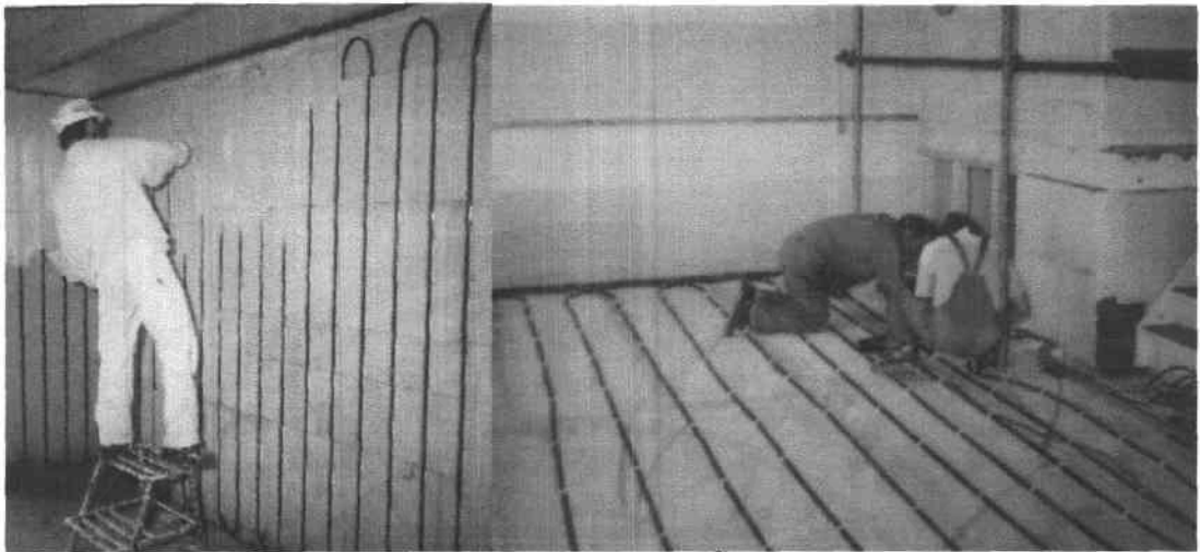
การเดินทาสีความร้อนไว้ในพื้นและผนัง
