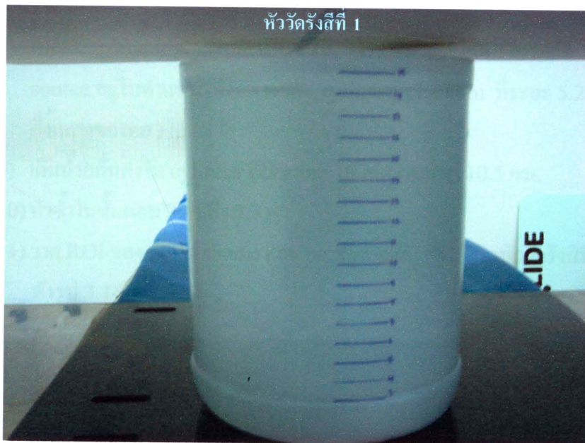
รูป 3.12 ตำแหน่งหัววัดรังสีที่วางบนขอบของ cylinder phantom ปอด
