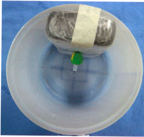
รูป 3.11 ตำแหน่ง point source ใน cylinder phantom ปอด
