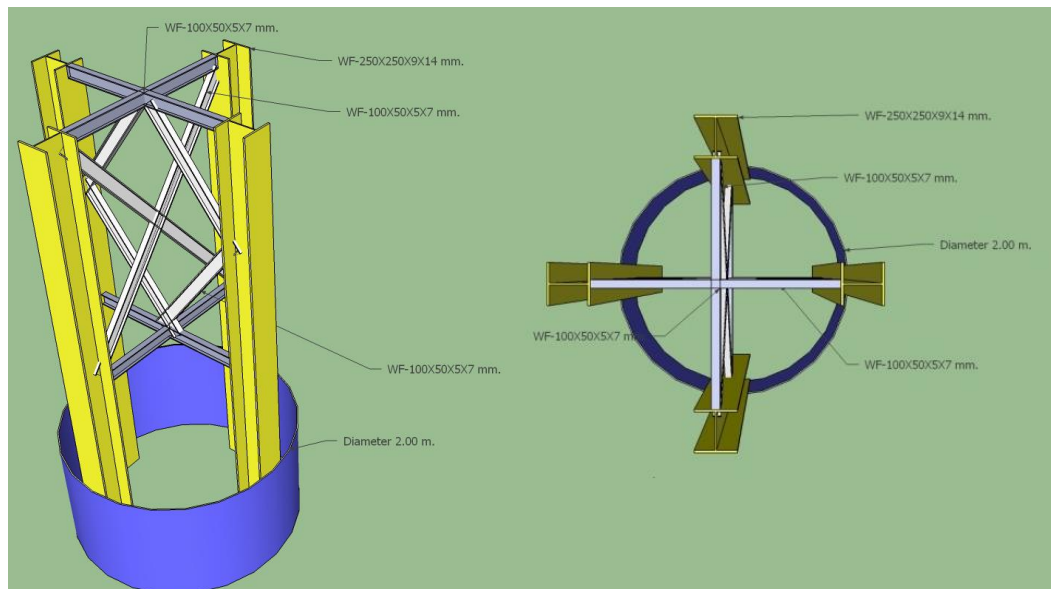
รูปที่ จ.4 แบบแปลน แบบขยายภายในเสาประกอบ เสากลมเดี่ยว เสากลมคู่ สามมิติ
