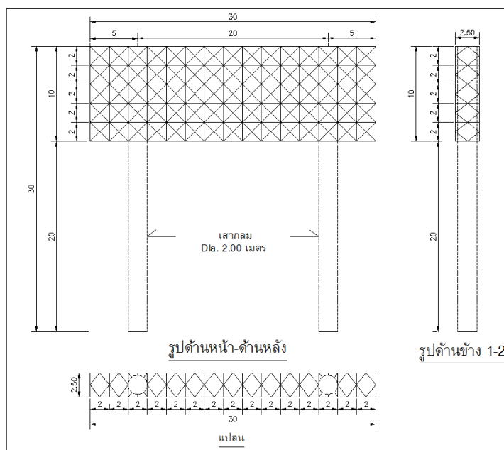
รูปที่ จ.2 แปลน รูปด้านหน้า ด้านหลัง ด้านข้าง 1 ด้านข้าง 2 เสากลมคู่
