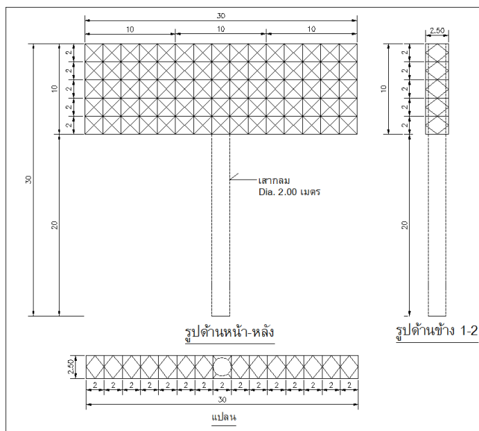
รูปที่ จ.1 แปลน รูปด้านหน้า ด้านหลัง ด้านข้าง 1 ด้านข้าง 2 เสากลมเดี่ยว
