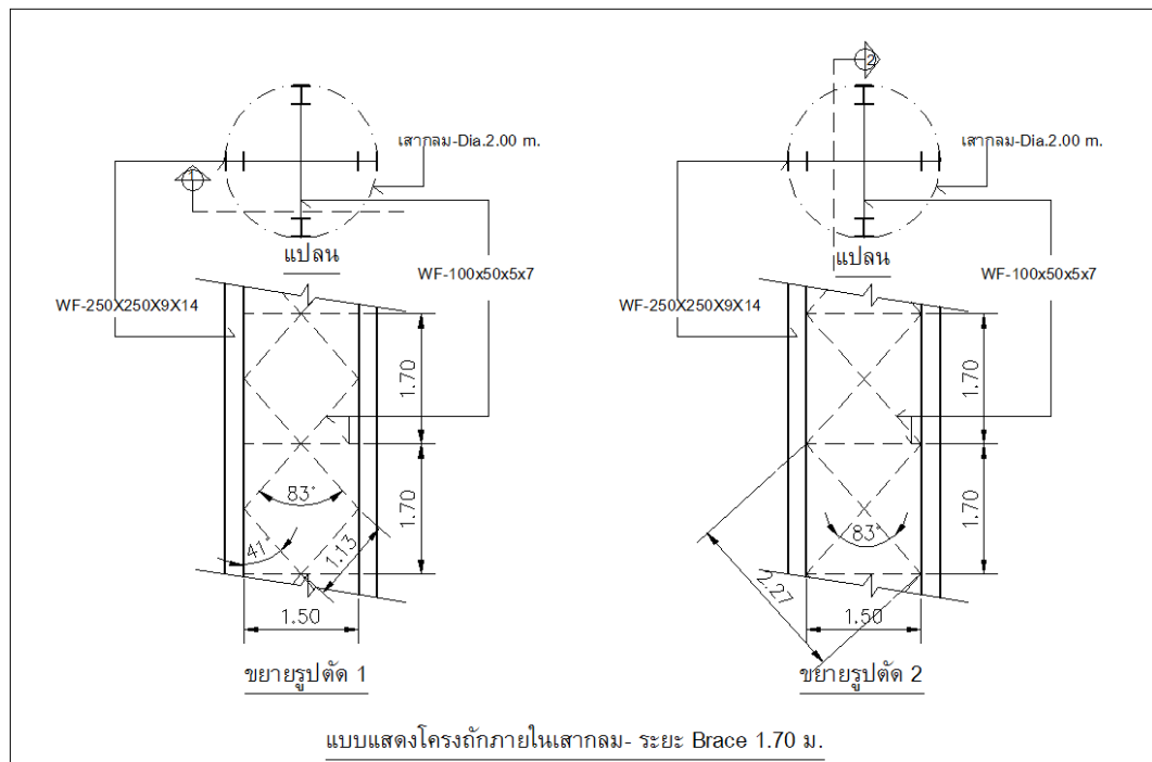
รูปที่ จ.3 แบบแปลน แบบขยายภายในเสาประกอบ เสากลมเดี่ยว เสากลมคู่
