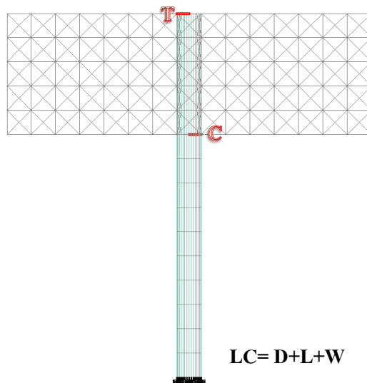
รูปที่ ง.1 แสดงตำแหน่งโครงข้อหมุนที่เกิดแรงในแนวแกนสูงสุด ลักษณะเสากลมเดี่ยว แรงลมกฎกระทรวง กรณีแรงลมตั้งฉากกับปีก
