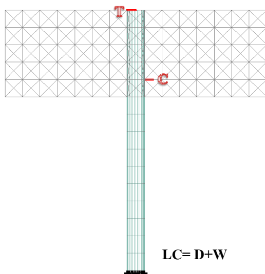
รูปที่ ง.3 แสดงตำแหน่งโครงข้อหมุนที่เกิดแรงในแนวแกนสูงสุด ลักษณะเสากลมเดี่ยว กลุ่มที่ 1 มยพ.1311-50 กรณีแรงลมตั้งฉากกับป้าย
