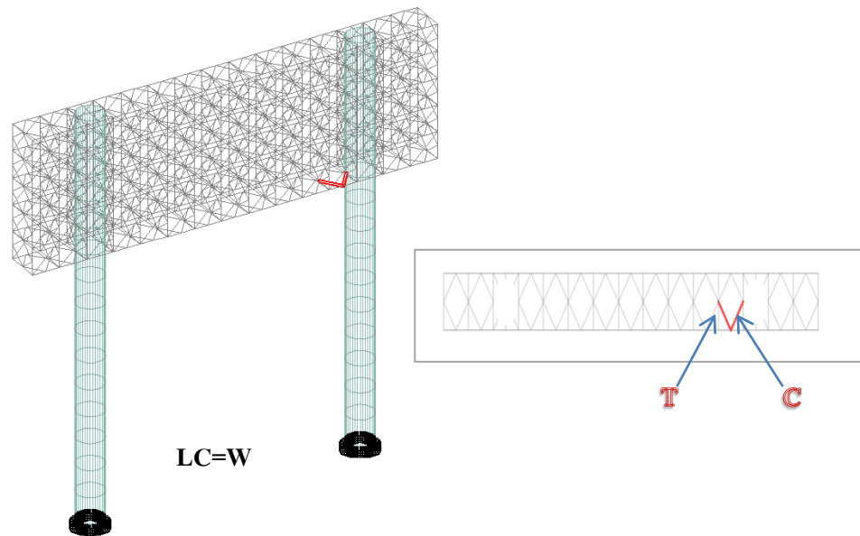
รูปที่ ง.7 แสดงตำแหน่งโครงข้อหมุนที่เกิดแรงในแนวแกนสูงสุด ลักษณะเสากลมคู่ กลุ่มที่ 1 กลุ่มที่ 2&4B กลุ่มที่ 3 และกลุ่มที่ 4A มยพ.1311-50 กรณีด้านขวาของป้ายชี้เข้าหาลม
