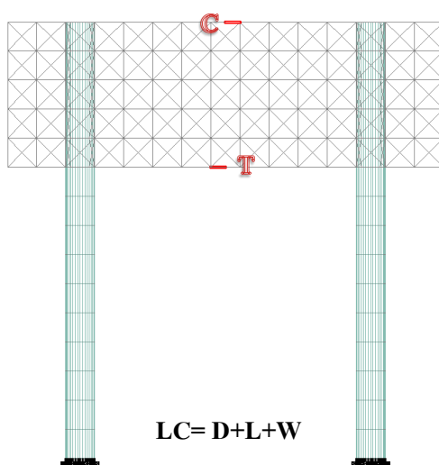
รูปที่ ง.2 แสดงตำแหน่งโครงข้อหมุนที่เกิดแรงในแนวแกนสูงสุด ลักษณะเสากลมคู่ แรงลมกฎกระทรวง กรณีแรงลมตั้งฉากกับปีก
