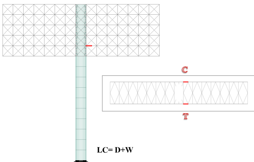
รูปที่ ง.4 แสดงตำแหน่งโครงข้อหมุนที่เกิดแรงในแนวแกนสูงสุด ลักษณะเสากลมเดี่ยว กลุ่มที่ 2 และกลุ่มที่ 4B กลุ่มที่ 3 กลุ่มที่ 4A มยพ.1311-50 กรณีแรงลมตั้งฉากกับป้าย
