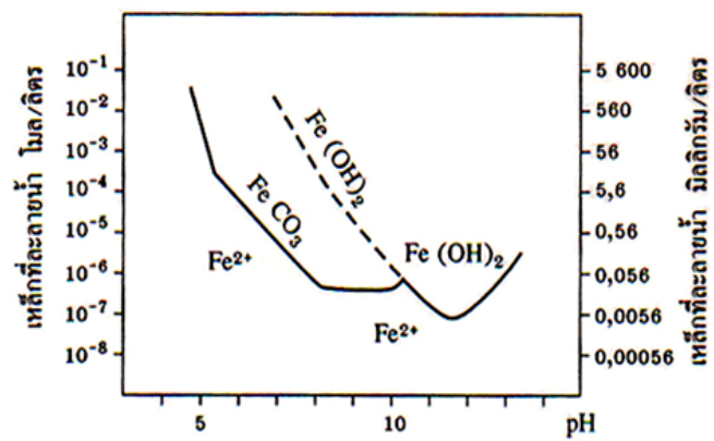
ภาพที่ 5 ความสัมพันธ์ pH กับความสามารถของเหล็กที่ละลายน้ำ
