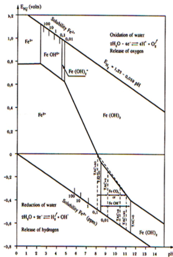
ภาพที่ 6 ค่า pH-potential ไดอะแกรมสำหรับเหล็ก
