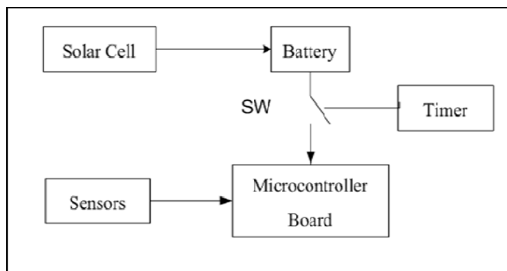
ภาพประกอบ 4-4 ภาพรวมของระบบรูปแบบที่ 4
