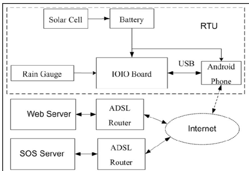
ภาพประกอบ 4-7 ระบบทำนายปริมาณน้ำฝนโดยใช้ฐานกฎ
